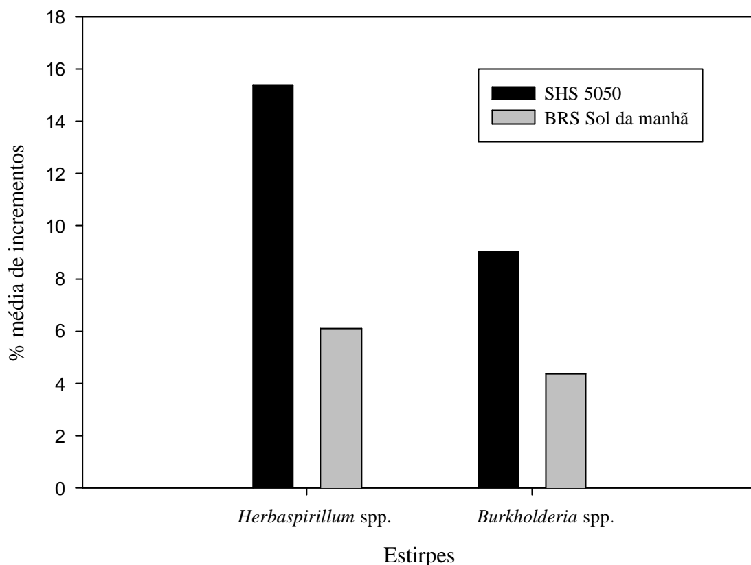
Figura 8. Médias de incrementos de biomassa seca dos tratamentos inoculados com Herbaspirillum spp. e Burkholderia spp. sobre a T20, na seleção em substrato não esterilizado, em milho híbrido SHS 5050 e milho variedade BRS Sol da Manhã.
