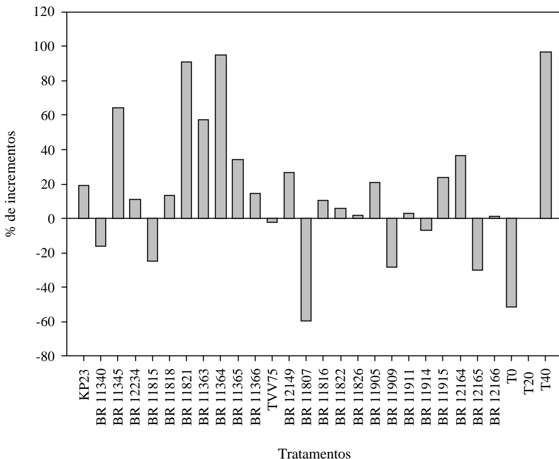
Figura 5. Valores relativos de biomassa seca dos tratamentos inoculados com Burkholderia spp. sobre a T20 (testemunha não inoculada e adubada com o equivalente a 20 kg ha -1 de N), na seleção em substrato esterilizado, em milho variedade BRS Sol da Manhã - Médias de 6 experimentos. Dados originais em anexo.
