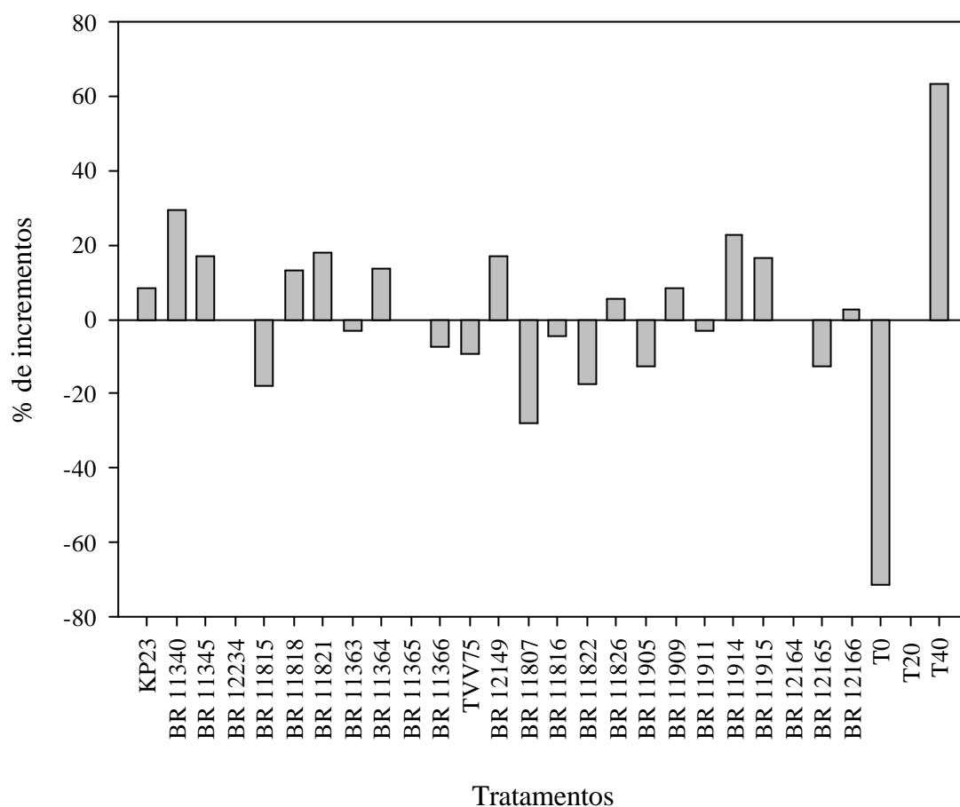
Figura 4. Valores relativos de biomassa seca dos tratamentos inoculados com Burkholderia spp. sobre a T20, (testemunha não inoculada e adubada com o equivalente a 20 kg ha -1 de N) na seleção em substrato esterilizado, em milho híbrido SHS 5050 - Médias de 6 experimentos. Dados originais em anexo.
