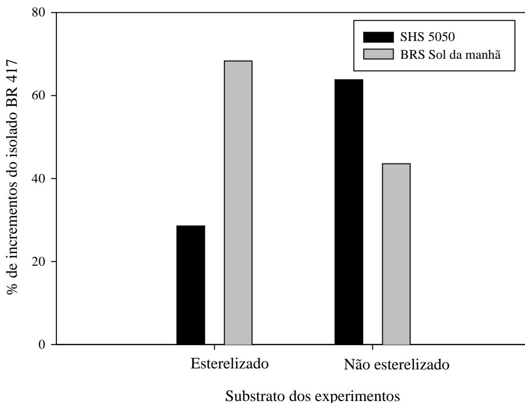
Figura 9. Incrementos de biomassa seca sobre a T20 (testemunha não inoculada e adubada com o equivalente a 20 kg ha -1 de N) de dois genótipos de milho inoculados com a estirpe Herbaspirillum seropedicae BR 11417 cultivados em substrato esterilizado e não esterilizado.
