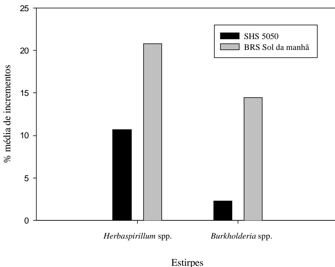
Figura 6. Médias de incrementos de biomassa seca dos tratamentos inoculados com Herbaspirillum spp. e Burkholderia spp. sobre a T20 (testemunha não inoculada e adubada com o equivalente a 20 kg ha -1 de N), na seleção em substrato esterilizado, em milho híbrido SHS 5050 e milho variedade BRS Sol da Manhã.
