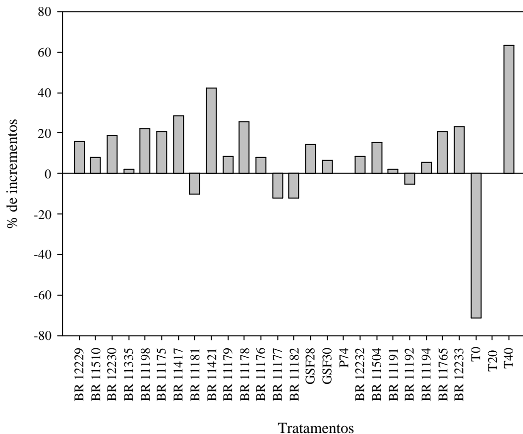
Figura 2. Valores relativos (%) de biomassa seca de parte aérea dos tratamentos inoculados com Herbaspirillum spp. sobre a T20 (testemunha não inoculada e adubada com o equivalente a 20 kg ha -1 de N), na seleção em substrato esterilizado, em milho híbrido SHS 5050 - Médias de 6 experimentos. Dados originais em anexo.
