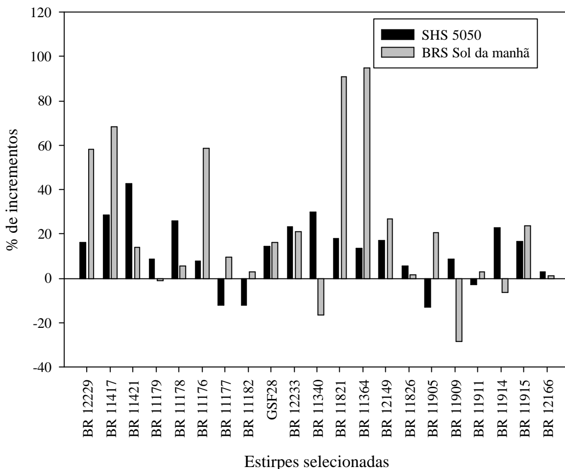
Figura 7. Valores relativos de biomassa seca dos tratamentos inoculados selecionados sobre a T20 (testemunha não inoculada e adubada com o equivalente a 20 kg ha -1 de N) em substrato esterilizado.
