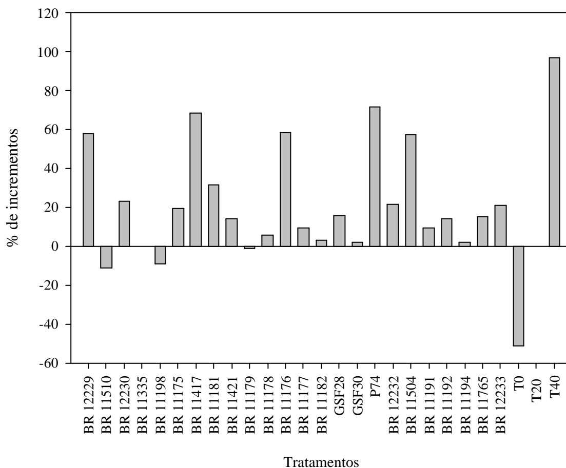
Figura 3. Valores relativos (%) de biomassa seca de parte aérea dos tratamentos inoculados com Herbaspirillum spp. sobre a T20 (testemunha não inoculada e adubada com o equivalente a 20 kg ha -1 de N), na seleção em substrato esterilizado, em milho variedade BRS Sol da Manhã - Médias de 6 experimentos. Dados originais em anexo.
