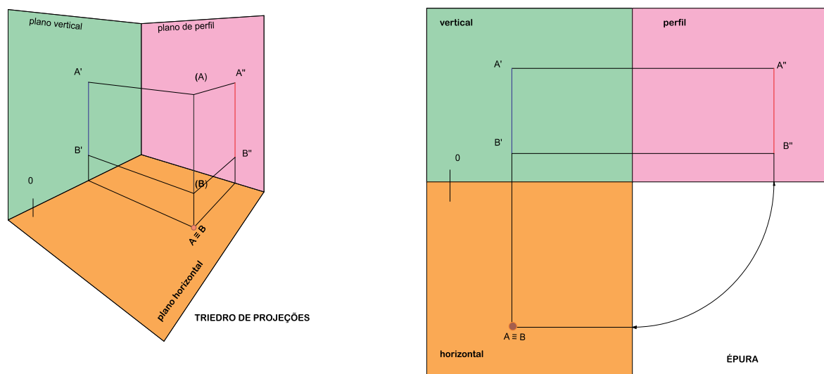
Figura 41- Reta vertical no primeiro diedro e sua Épura.
