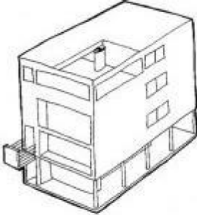
Figura 7- Perspectiva isométrica (cilíndrica ou paralela) da casa Citrohan Mark II de Le Corbusier. As linhas do desenho são paralelas.
