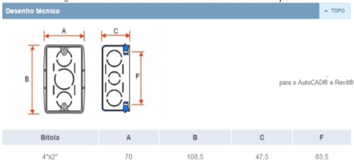
Figura 12 – Desenho técnico de caixa de luz. Vistas frontal e lateral esquerda.
