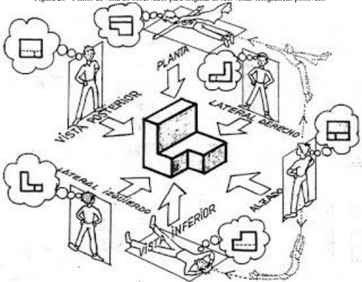
Figura 26 - Pontos de vista do observador para originar as seis vistas ortográficas possíveis.
