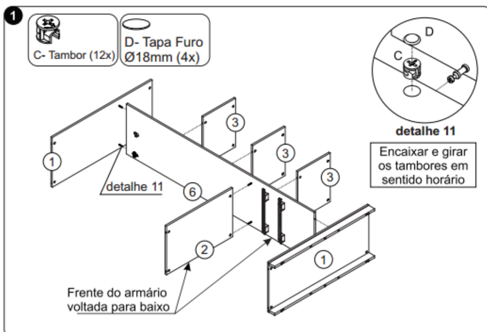
Figura 15- Perspectiva explodida para detalhamento da montagem do armário apresentado na figura 14. Detalhe de manual online da Tok&Stok.
