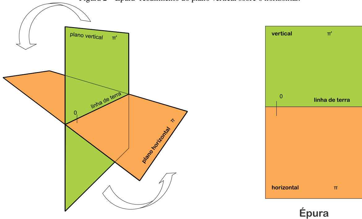
Figura 2 – Épura- rebatimento do plano vertical sobre o horizontal.
