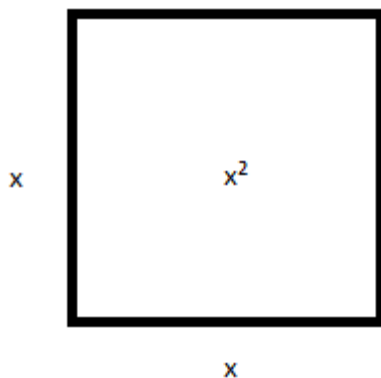
Figura 1 Quadrado de área x^2
