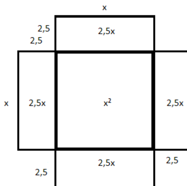
Figura 2 Figura de área x^2 + 10x
