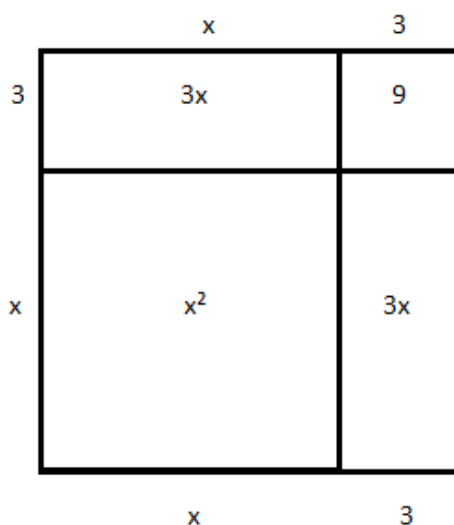
Figura 18 Quadrado de área x^2 + 6x + 9
