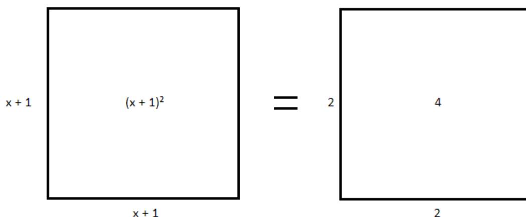
Figura 20 Igualdade (x+1)^2 = 2^2
