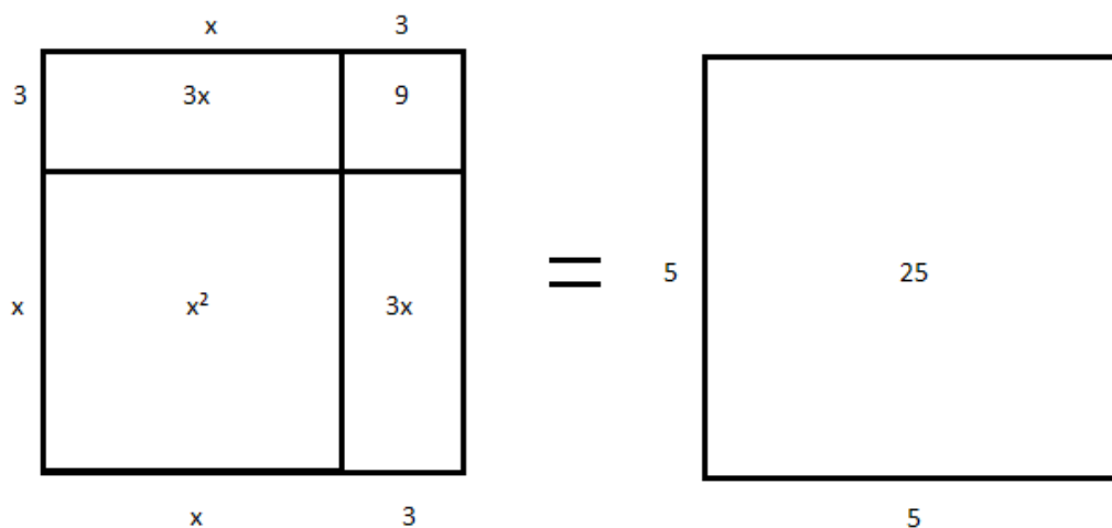
Figura 19 Igualdade (x + 3)^2 = 5^2
