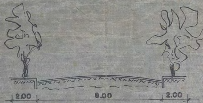
CORTE TRANSVERSAL DAS RUAS ESCALA 1 : 2.000
