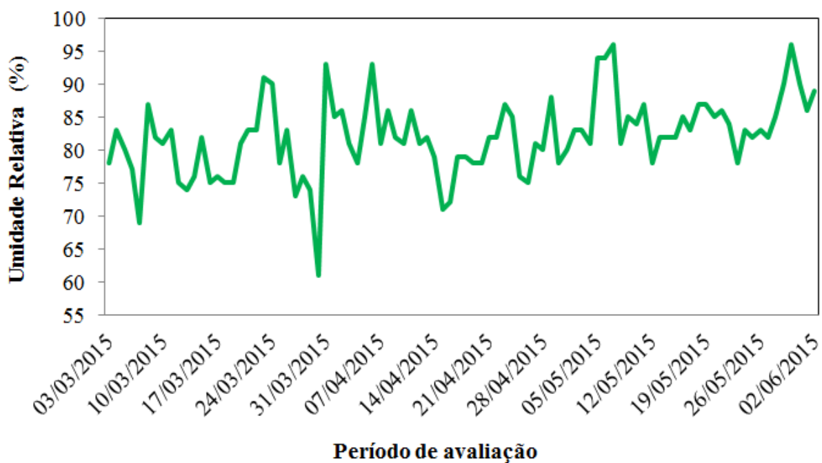
Figura 5. Umidade relativa do ar registrada no período de 03 de março a 02 de junho de 2015 pela Estação Meteorológica Convencional de Viçosa – MG (UFV)
