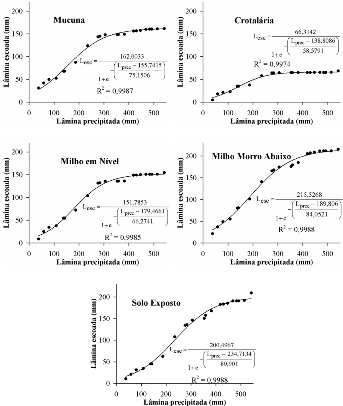
Figura 10. Lâminas totais escoadas acumuladas (mm) em função das lâminas totais precipitadas acumuladas (mm) para os tratamentos Mucuna, Crotalária, Milho em Nível, Milho Morro a Baixo e Solo Exposto.
