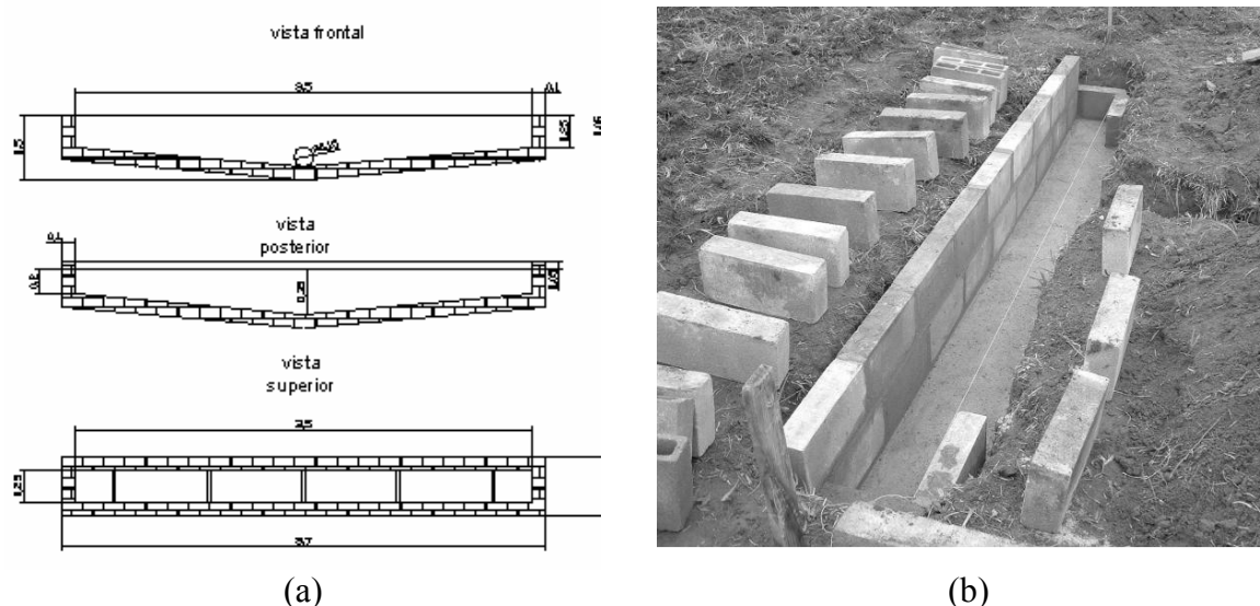
Figura 3. Detalhes construtivos das calhas coletoras de enxurradas construídas para o estudo de perdas de solo e água.
