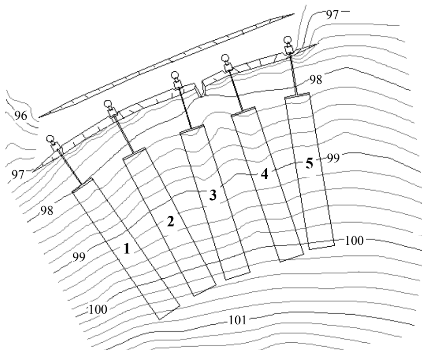
Figura 2. Disposição das parcelas experimentais com os tratamentos Mucuna (1), Milho em Nível (2), Milho Morro a Baixo (3), Crotalária (4) e Solo Exposto (5).
