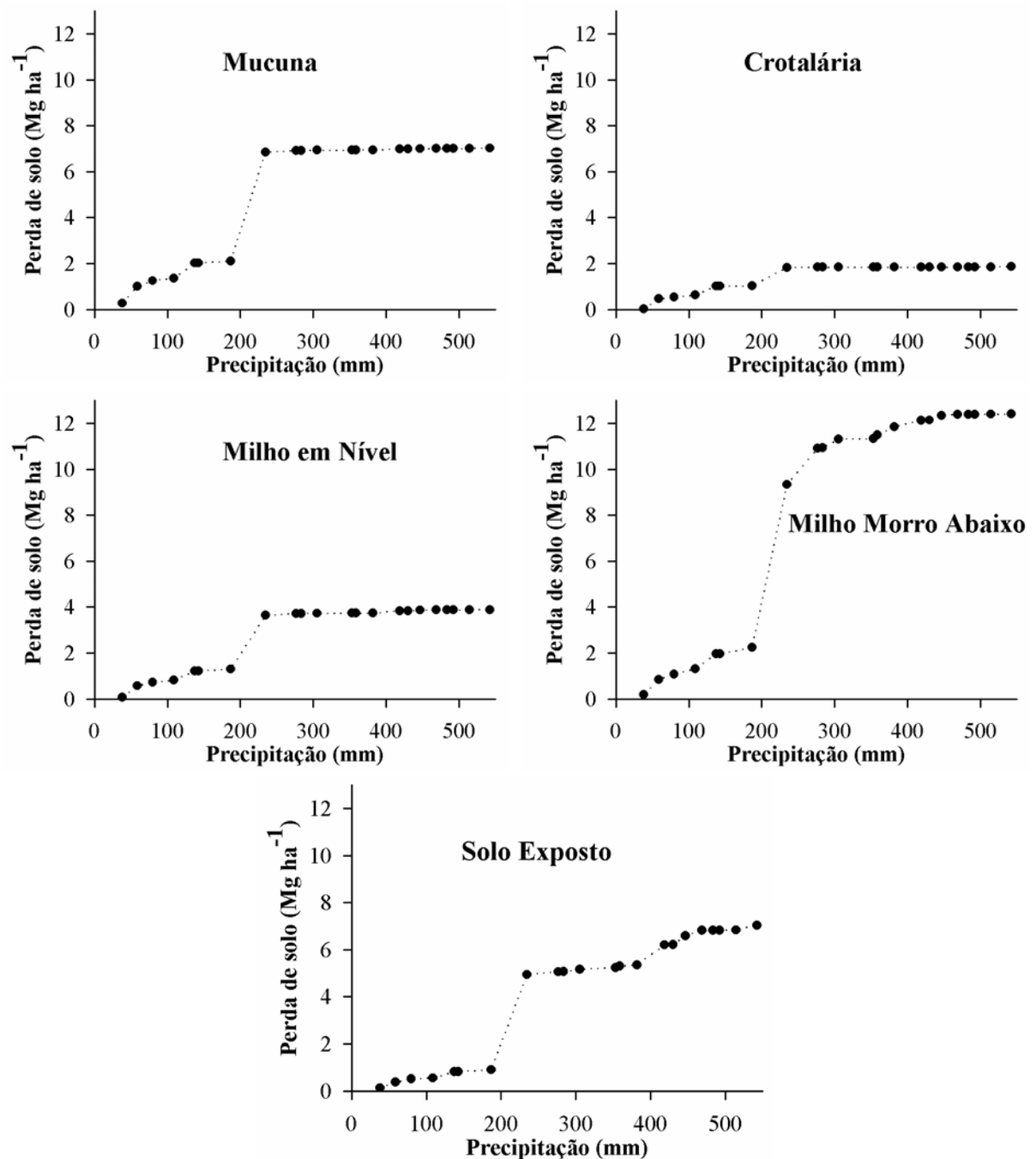
Figura 11. Perdas acumuladas de solo, em função das lâminas precipitadas acumuladas, para os tratamentos Mucuna, Crotalária, Milho em Nível, Milho Morro a Baixo e Solo Exposto
