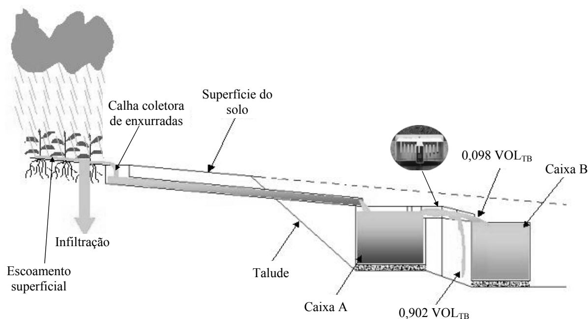
Figura 4. Esquema do funcionamento do conjunto das estruturas utilizadas nas coletas de perdas de solo e água.
