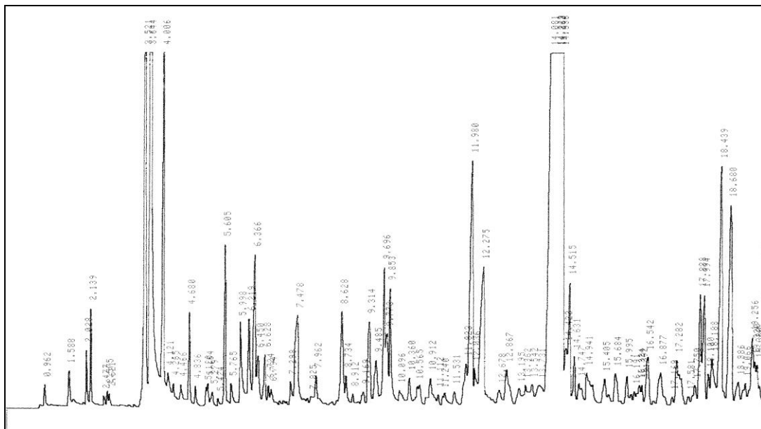
Figura 11 - Cromatograma da amostra do retido do processo a 25°C com a membrana de EPDM e extração por SPME.
