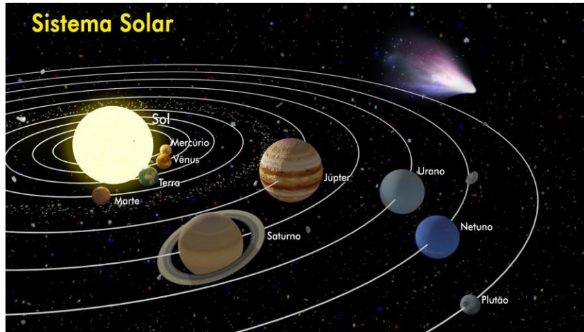
Figura 7 – Órbitas elípticas dos planetas.
