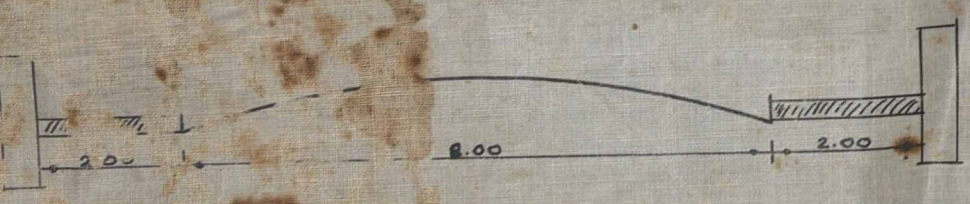
PERFIL TRANSVERSAL - ESCALA: 1/100
