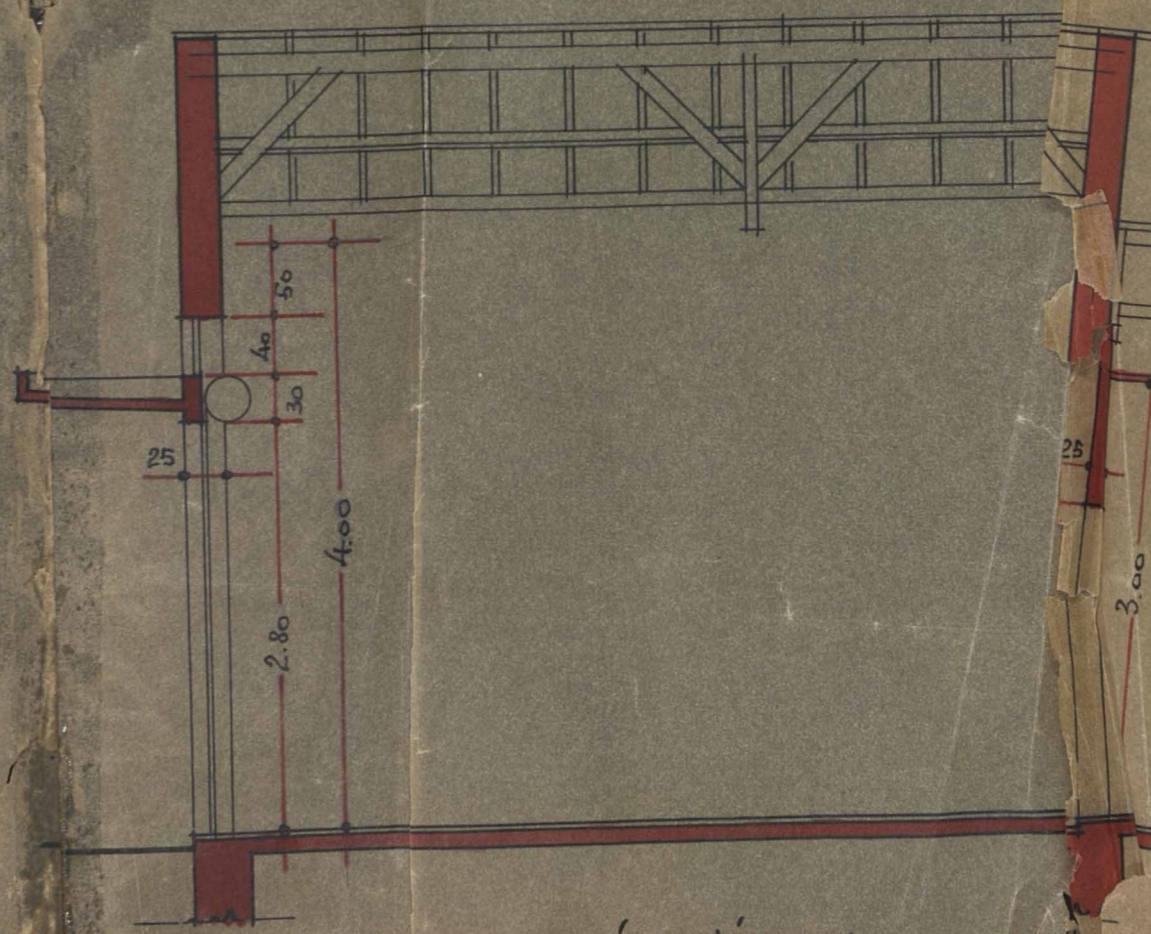
corte longitudinal esc. 1:50
