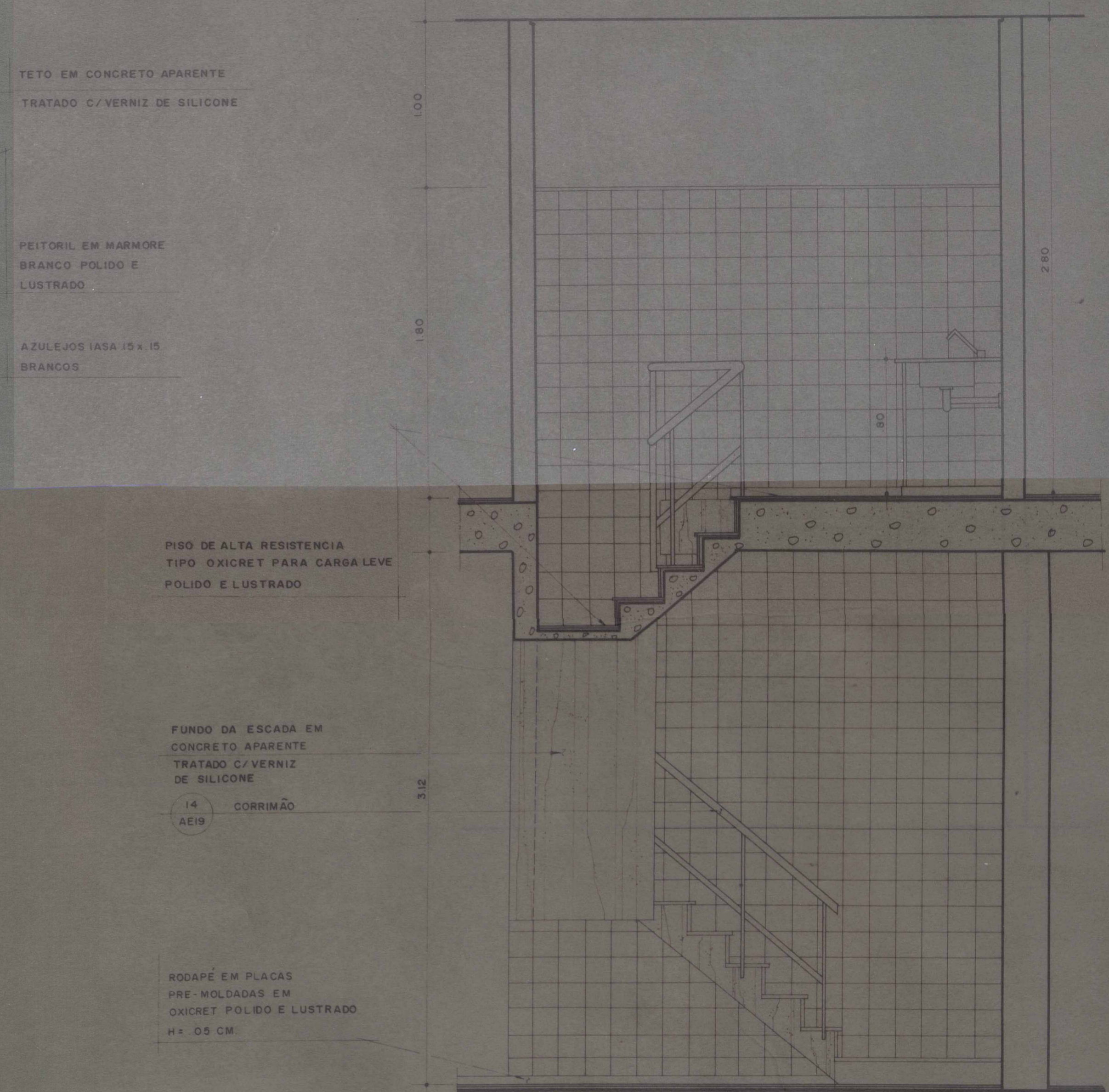
COPA 02 - CANTINA - DEPÓSITO CORTE DD ESC. 1/20
