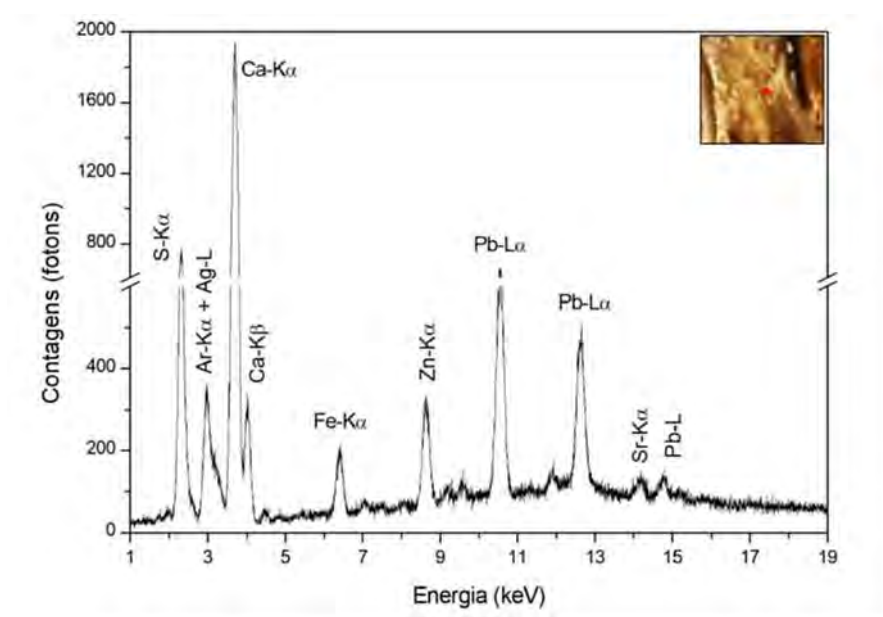
Figura 79. Espectro de XRF obtido na camada de preparação da escultura do Rei Davi. Fonte: LIETA/UERJ, 2021.
