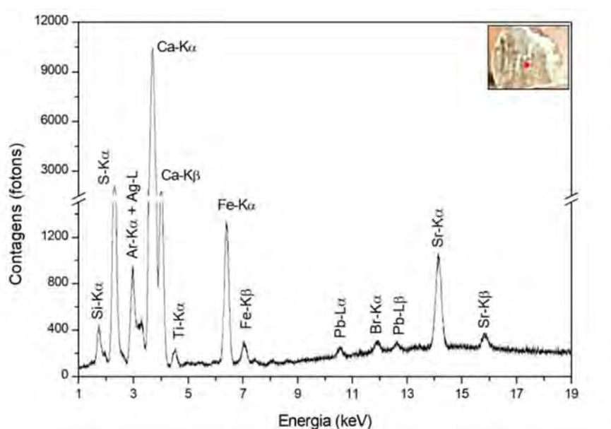
Figura 89. Espectro de XRF obtido na madeira da escultura de Betsabá. Fonte: LIETA/UERJ, 2021.
