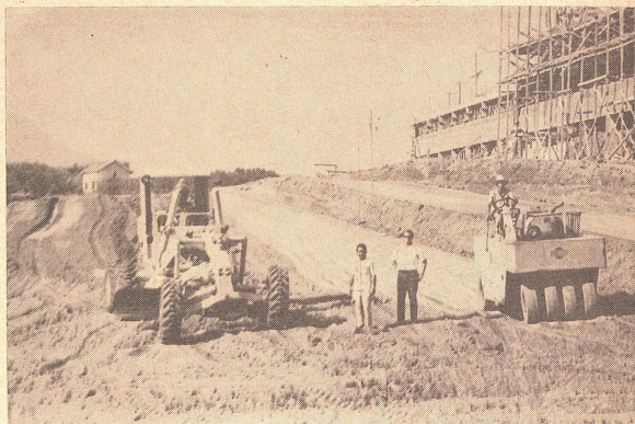
Andamento das obras da CESP, na terraplanagem da fábrica de cigarros Santa-Cruz.
