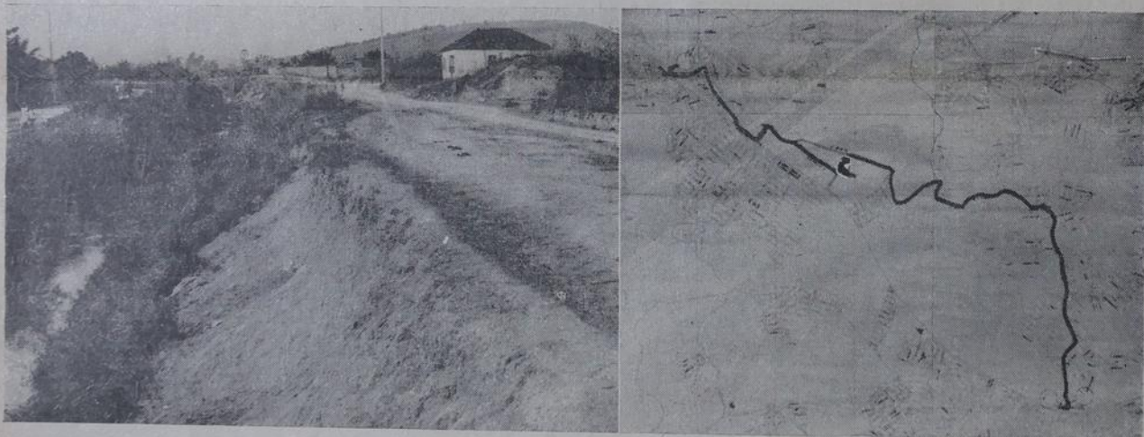
A foto mostra o rio que causava a erosão em quase toda a extensão da estrada — que a planta mostra, — hoje terraplenada
