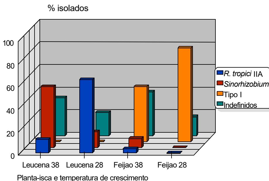
Figura 7: Distribuição dos isolados dentro das espécies definidas por ARDRA, de acordo com a planta-isca e temperatura de crescimento utilizada para recuperação do rizóbio do solo.
