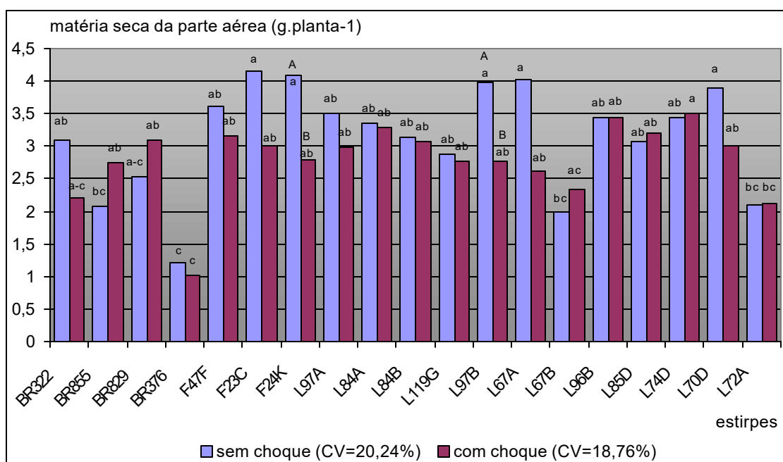
Figura 3: Produção de matéria seca da parte aérea de feijoeiro, cv Carioca 80, inoculado com diferentes estirpes de rizóbio. Avaliação aos 43DAE, 9 dias após um período de choque térmico. Valores médios de 4 repetições. Letras diferentes contrastam pelo teste de Tukey ( P=0,05 ). Diferenças entre as estirpes estão indicadas pelas letras minúsculas, e o efeito do tratamento para cada estirpe pelas letras maiúsculas.
