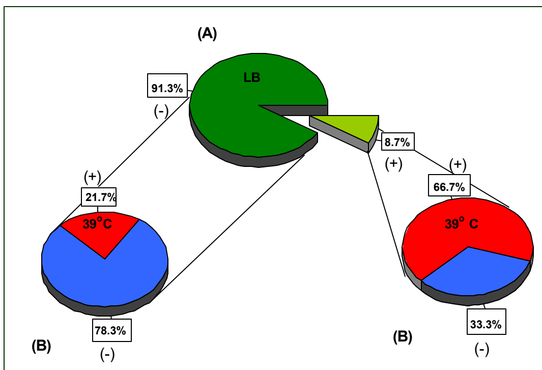
Figura 3: Porcentagem de isolados de Phaseolus vulgaris apresentando crescimento positivo(+) ou negativo (-) em meio LB (A) e tolerância in vitro temperaturas elevadas avaliada pela capacidade de crescer (+) ou não (-) em meio YMA a 39°C (B) .
