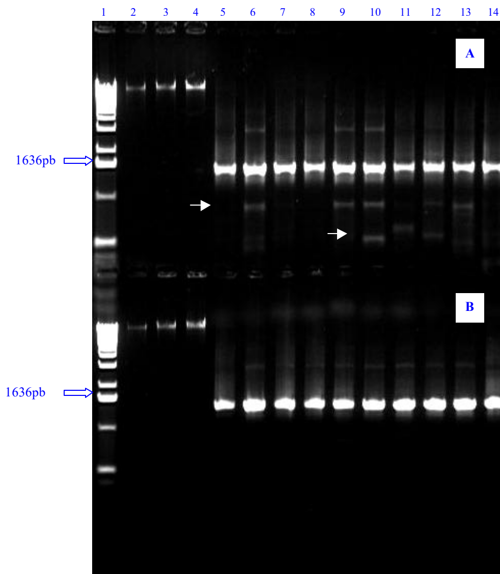
Figura 2: Reação de amplificação do DNA obtido através do método da fervura ( A ) e da lise alcalina ( B ) mostrando a ocorrência de reações inespecíficas em (A) para amostras com padrão semelhante de concentração do produto da amplificação. 1: marcador de peso molecular (1Kb); 2 a 4: concentrações crescentes de DNA :10, 20 e 40 ug.ul -1 ; 5: BR5410; 6 – BR322; 7 – GMI9023; 8 – A. rhizogenes ; 9 – BR10026; 10 – BR10055; 11 – BR112; 12 – BR7411; 13 – BR78901; 14 – BR111.
