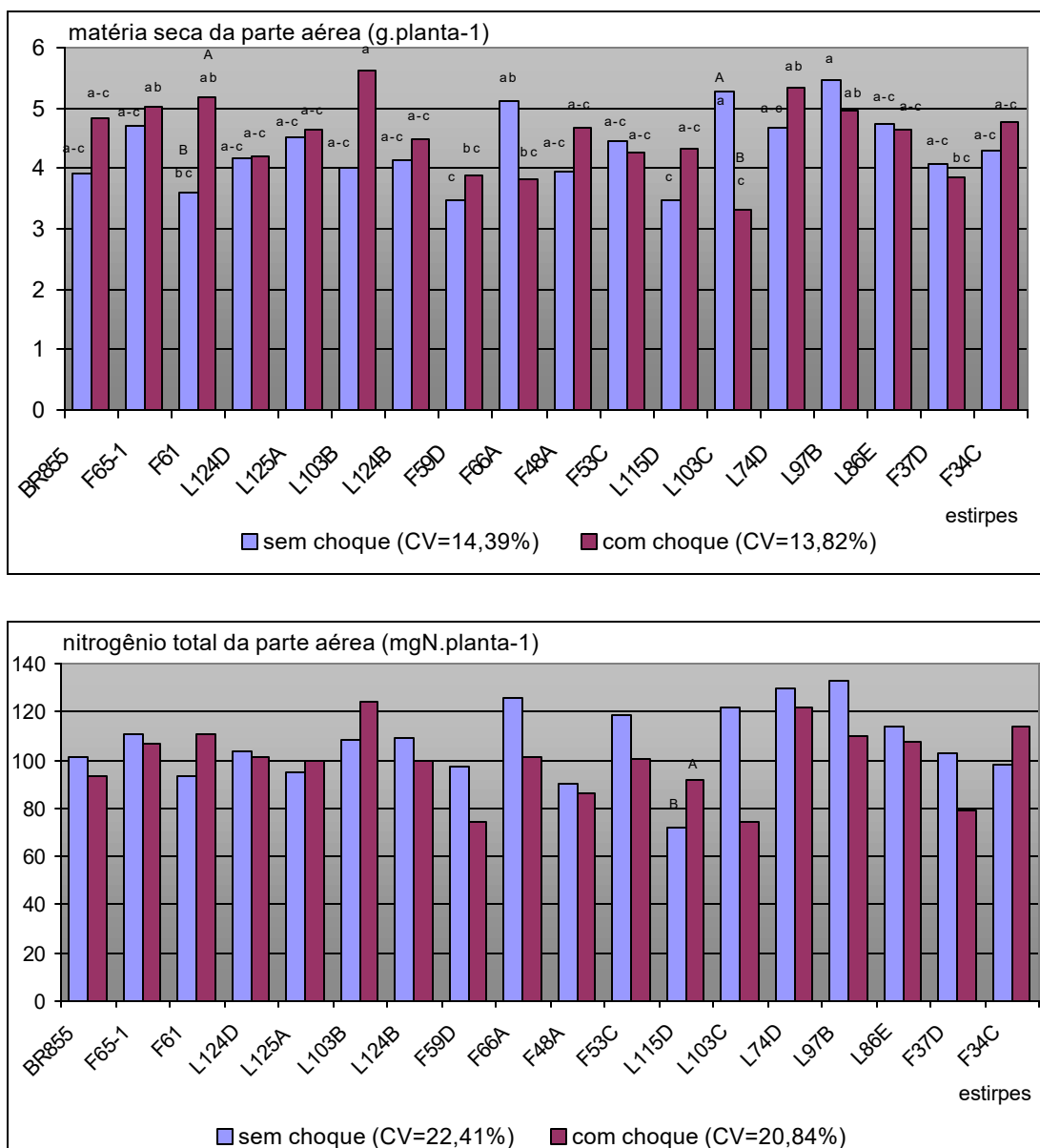
Figura 6: Produção de matéria seca e nitrogênio total da parte aérea de feijoeiro, cv Carioca 80, inoculado com diferentes estirpes de rizóbio. Avaliação aos 44 DAE, 6 dias após um período de choque térmico. Valores médios de 4 repetições. Letras diferentes contrastam pelo teste de Tukey ( P=0,05 ). Diferenças entre as estirpes estão indicadas pelas letras minúsculas, e o efeito do tratamento para cada estirpe pelas letras maiúsculas.
