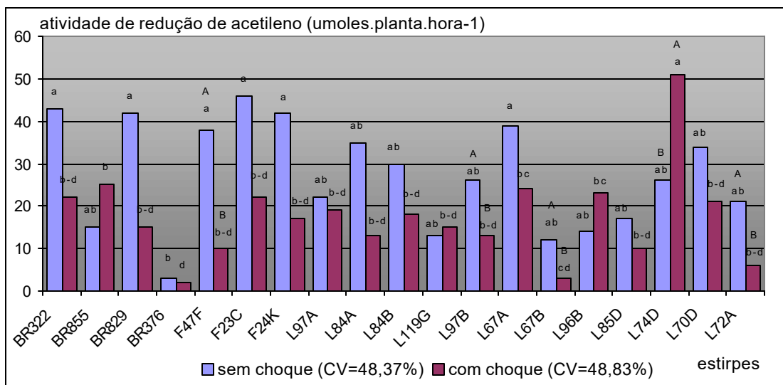
Figura 2: Atividade de redução de acetileno das raízes noduladas de feijoeiro, cv Carioca 80, inculadas com diferentes estirpes de rizóbio. Avaliação aos 43DAE, 9 dias após um período de choque térmico. Valores médios de 4 repetições. Letras diferentes contrastam pelo teste de Tukey ( P=0,05 ). Diferenças entre as estirpes estão indicadas pelas letras minúsculas, e o efeito do tratamento para cada estirpe pelas letras maiúsculas.
