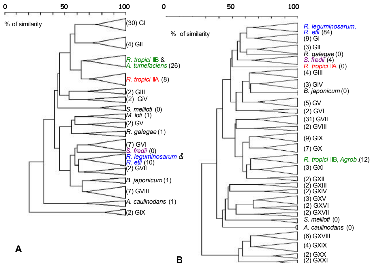
Figura 5: Análise de agrupamento mostrando a distribuição de 124 isolados recuperados de feijoeiro ( Phaseolus vulgaris ) crescido a temperatura ambiente (A) e de 219 isolados recuperados a temperaturas elevadas (B) . Análise de agrupamento pelo método UPGMA e o coeficiente de similaridade S_{SM} (simple matching). Entre parêntesis está indicado o número de isolados pertencentes a cada agrupamento.
