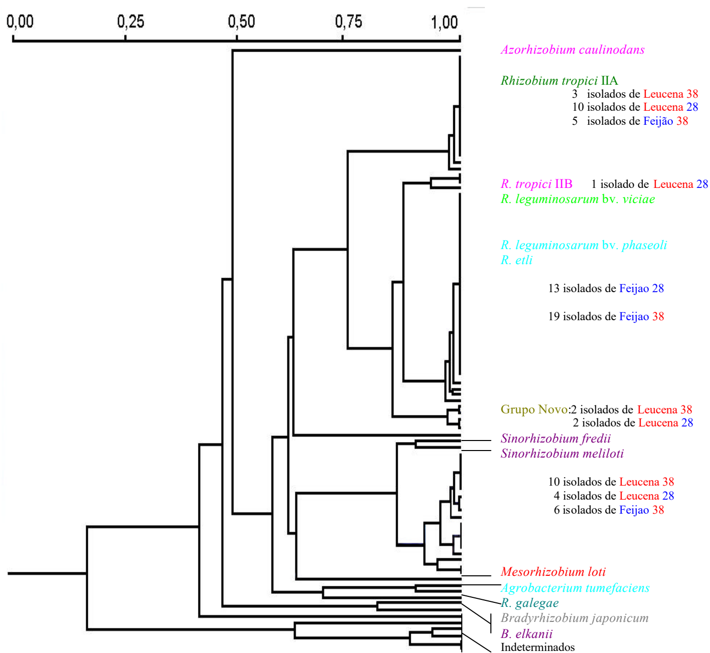
Figura 6: Dendrograma de agrupamento dos 83 isolados representativos dos grupos fenotípicos obtidos no Capítulo I. As distâncias foram derivadas da fração de fragmentos de digestão do DNAr 16S compartilhados (DICE) conforme descrito em Material e Métodos.
