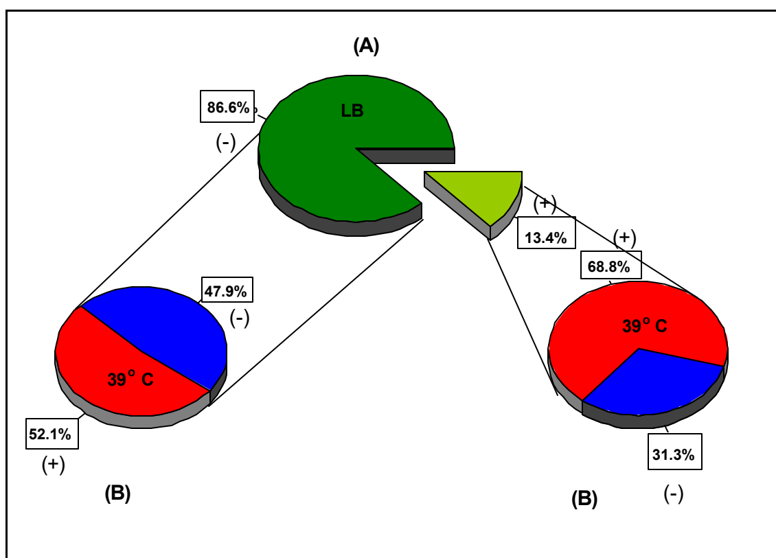
Figura 2: Porcentagem de isolados de Leucaena leucocephala apresentando crescimento positivo (+) ou negativo (-) em meio LB (A) e tolerância in vitro temperaturas elevadas avaliada pela capacidade de crescer (+) ou não (-) em meio YMA a 39°C (B) .
