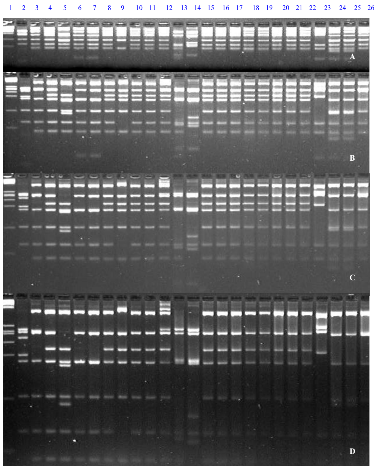
Figura 5: Padrões de restrição do DNAr 16S, obtidos pela incubação com a enzima Hae III. Sequência de fotos dos géis (Metaphor-FMC a 3,5%, 120V) de restrição após 1 (A), 2 (B) e 4 (C) e 6 (D) horas de corrida. Amostras conforme Figura 4. Padrão de peso molecular PhiX174 RF DNA Hae III Digest, BioLabs.
