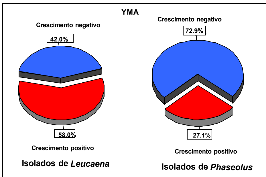
Figura 1: Porcentagem de isolados de feijoeiro ( Phaseolus vulgaris ) ou leucena ( Leucaena leucocephala ) que apresentaram crescimento positivo ou negativo em meio YMA (Vincent, 1970) a 39°C.
