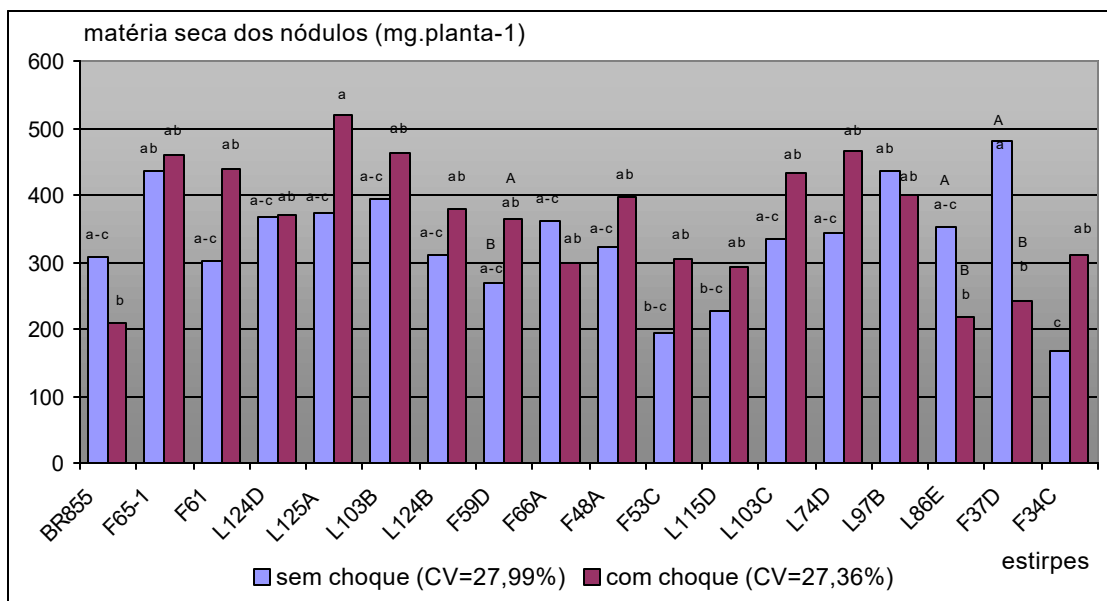
Figura 4: Produção de matéria seca nos nódulos de feijoeiro, cv Carioca 80, inoculado com diferentes estirpes de rizóbio. Avaliação aos 44 DAE, 6 dias após um período de choque térmico. Valores médios de 4 repetições. Letras diferentes contrastam pelo teste de Tukey ( P=0,05 ). Diferenças entre as estirpes estão indicadas pelas letras minúsculas, e o efeito do tratamento para cada estirpe pelas letras maiúsculas.
