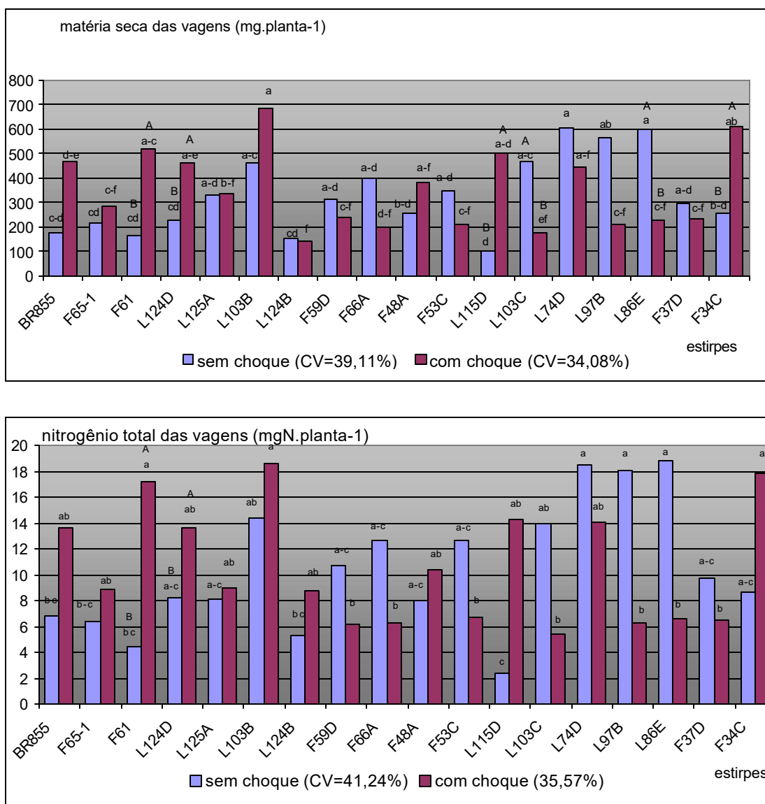
Figura 5: Produção de matéria seca e nitrogênio total das vagens de feijoeiro, cv Carioca 80, inculado com diferentes estirpes de rizóbio. Avaliação aos 44 DAE, 6 dias após um período de choque térmico. Valores médios de 4 repetições. Letras diferentes contrastam pelo teste de Tukey ( P=0,05 ). Diferenças entre as estirpes estão indicadas pelas letras minúsculas, e o efeito do tratamento para cada estirpe pelas letras maiúsculas.
