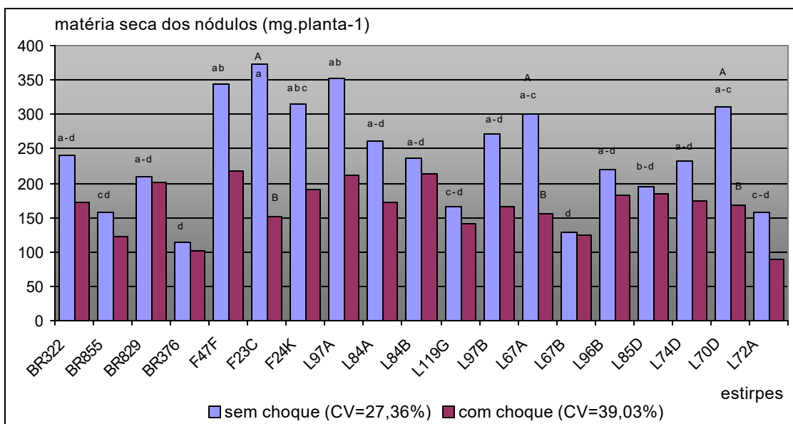
Figura 1: Produção de matéria seca nos nódulos de feijoeiro, cv Carioca 80, inculado com diferentes estirpes de rizóbio. Avaliação aos 43DAE, 9 dias após um período de choque térmico. Valores médios de 4 repetições. Letras diferentes contrastam pelo teste de Tukey ( P=0,05 ). Diferenças entre as estirpes estão indicadas pelas letras minúsculas, e o efeito do tratamento para cada estirpe pelas letras maiúsculas.
