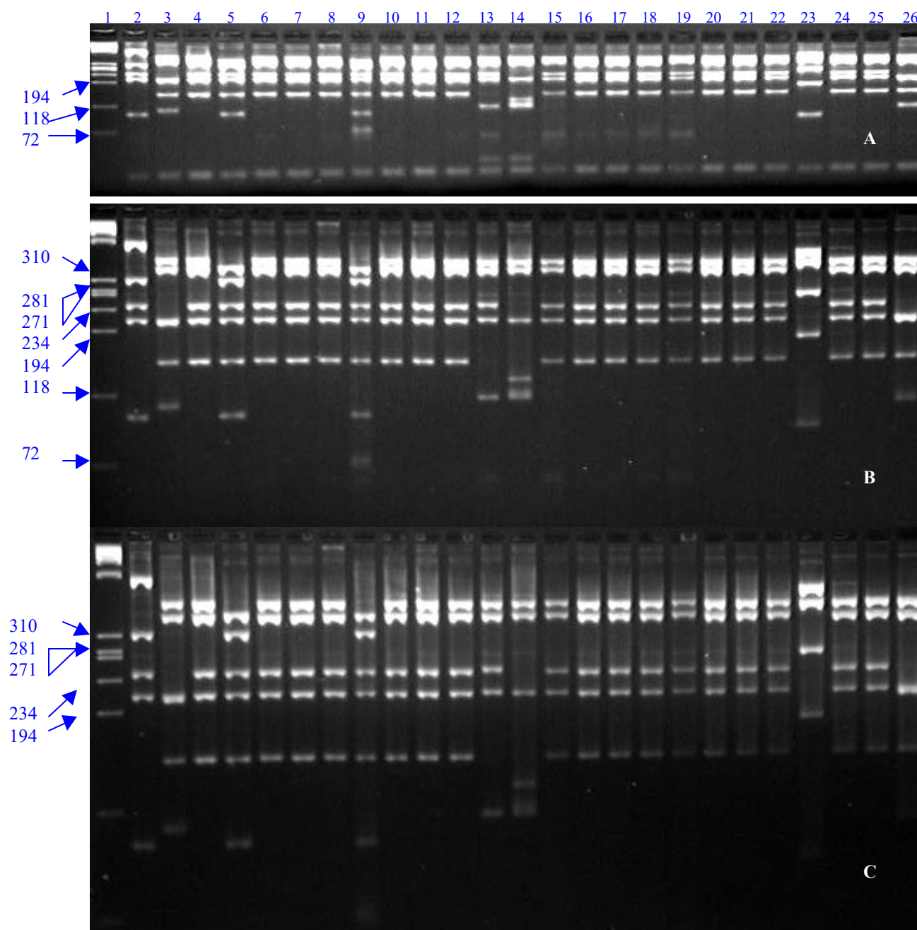
Figura 4: Padrões de restrição do DNAr 16S, obtidos pela incubação com a enzima Dde I. Fotos dos géis (Metaphor-FMC a 3,5%, 120V) após 2 (A), 4 (B) e 6 (C) horas de corrida. Observar o desaparecimento das bandas comparando com o padrão de peso molecular (PhiX174 RF DNA Hae III Digest, BioLabs) corredor (1). (2): A. caulinodans -BR5410; (3): R. tropici IIA-BR10016; (3): R. tropici IIB-BR322; (4) A. tumefaciens -GMI9023; (5) R. etli -BR10026; (6) R. leguminosarum bv. phaseoli -BR10052; (7) R. leguminosarum bv. viciae -BR620; (8) R. galegae -BR10055; (9) S. fredii -BR112; (10) S. meliloti -BR7410; (11) M. loti -BR7801; (12) B. japonicum -BR111; (13) B. elkanii -BR29; (14 a 26) isolados de Leucaena L1 a L13.
