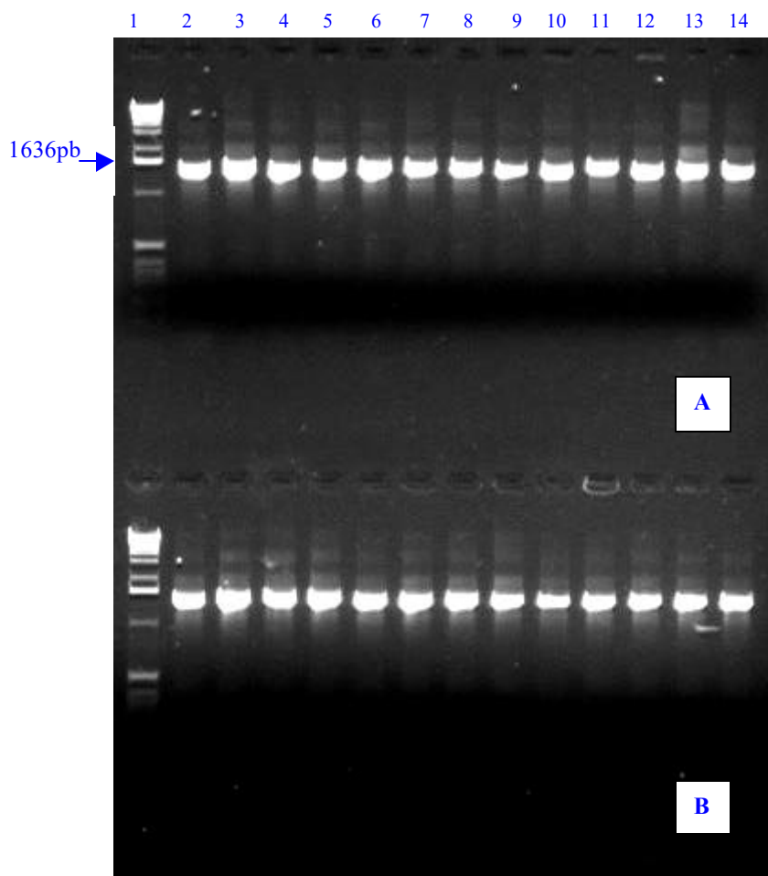
Figura 3: Amplificação do DNA dos isolados de leucena e feijoeiro extraído pelo método de lise alcalina. (A) Amostras 2 a 9: isolados de leucena segundo numeração sequencial de L26 a L34; amostras 10 a 14: isolados de feijoeiro F35 a F39. (B) Amostras 2 a 14: isolados de feijoeiro: F39 a F51. O padrão de peso molecular utilizado (1) foi o 1Kb DNA ladder (GIBCO BRL).
