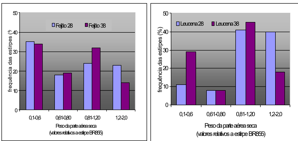
Figura 6: Eficiência na fixação de nitrogênio em simbiose com o feijoeiro dos isolados obtidos a partir de feijoeiro e leucena, em duas temperaturas de incubação das plantas, medida em valores relativos a estirpe BR855.
