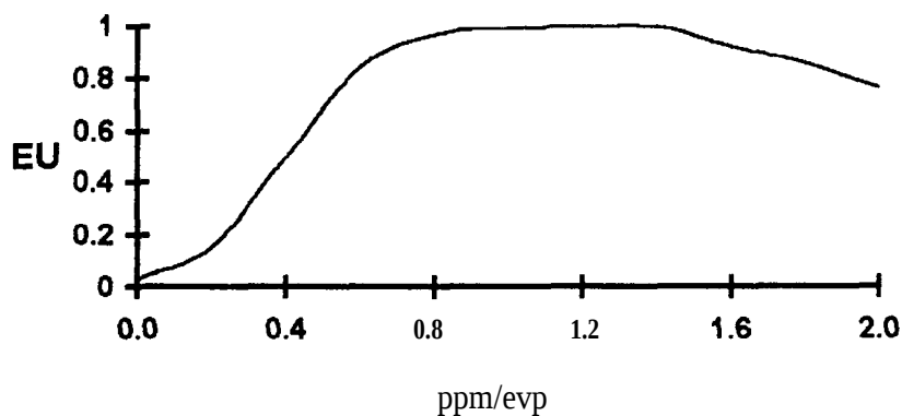
Figura 2: Efeito da relação precipitação/evapotranspiração sobre a taxa de decomposição da M.O. do solo (Parton et al., 1987).
