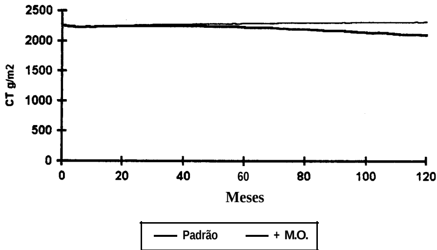
Figura 19: Resposta da variável Carbono total (CT) a adição de M.O.
