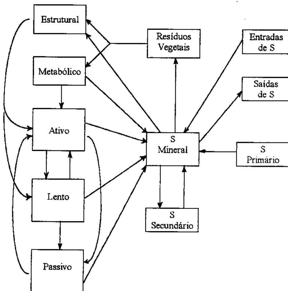
Figura 8: Ciclo do enxofre (Parton et al. , 1988).
