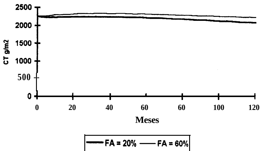
Figura 18: Resposta da variável Carbono total (CT) ao aumento da Fração argila (FA) do solo.
