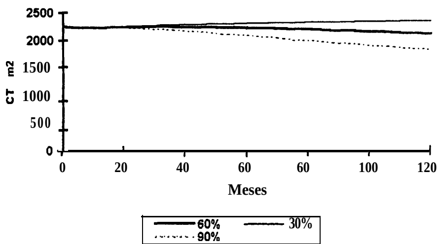
Figura 16: Resposta da variável Carbono total (CT) nas simulações variando-se os valores de Carbono alocado na parte aérea.
