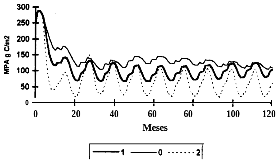
Figura 17: Resposta da variável Massa de parte aérea (MPA) nas simulações variando-se os valores de Fator de senescência.
