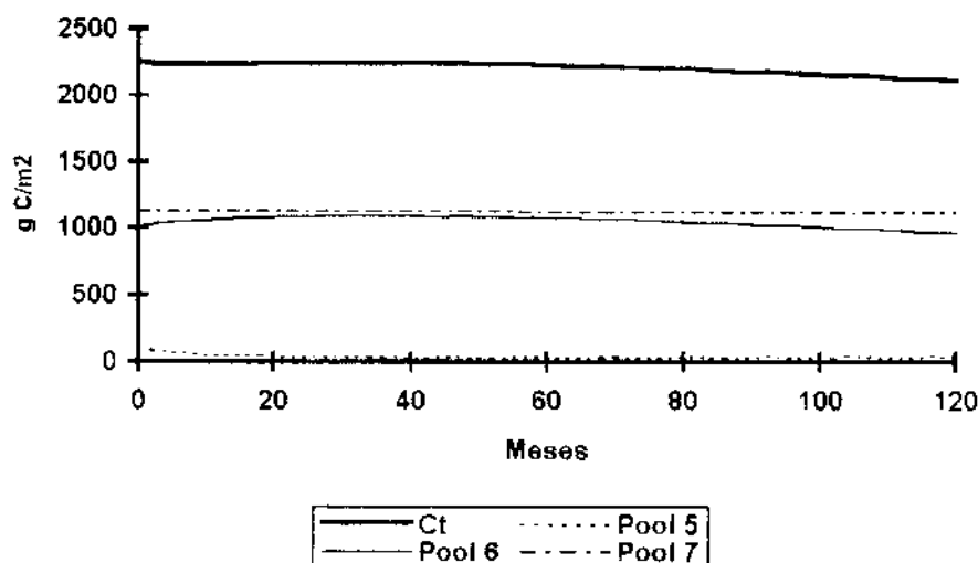
Figura 10: Resposta das variáveis Carbono total (CT), "Pool" 5, "Pool" 6 e "Pool" 7 nas simulações com os valores iniciais inalterados.
