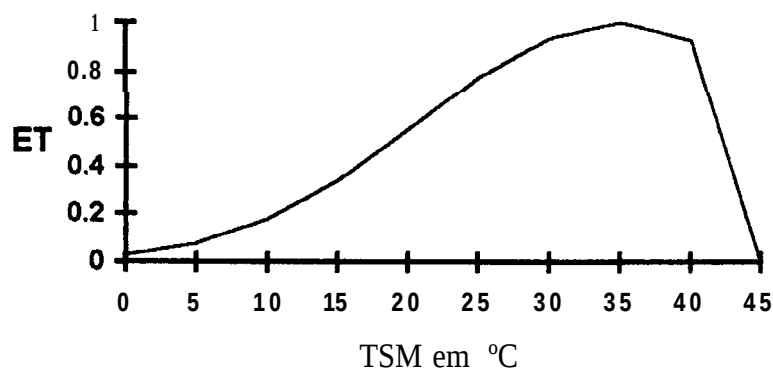
Figura 3: Efeito da temperatura sobre a taxa de decomposição da M.O. do solo (Barton et al., 1987).
