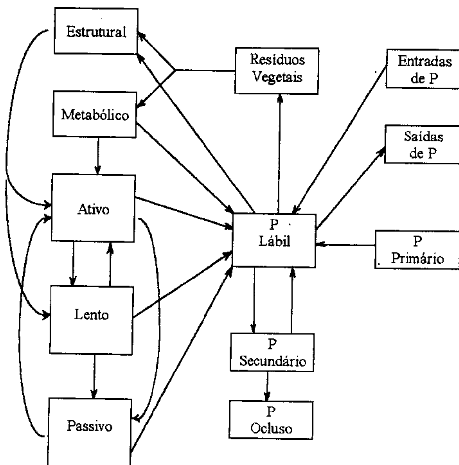
Figura 6: Ciclo do fósforo (Parton et al. , 1988).
