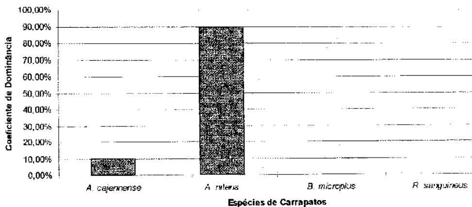
Gráfico 5: Coeficiente de Dominância entre espécies de carrapatos para Equus caballus examinados na Zona Fisiográfica de Resende, estado do Rio de Janeiro, em 1997.
