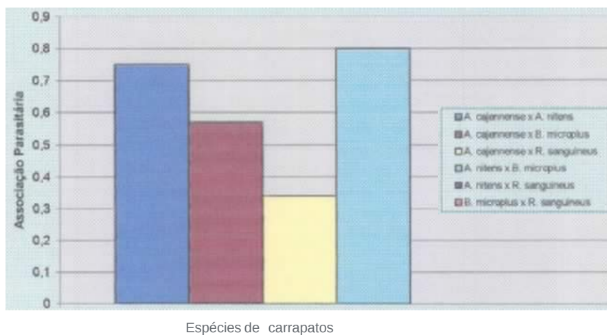
Gráfico 8: Associação Parasitária entre quatro espécies de carrapatos parasitos de seis espécies de hospedeiros na Zona Fisiográfica de Resende, estado do Rio de Janeiro, em 1997.
