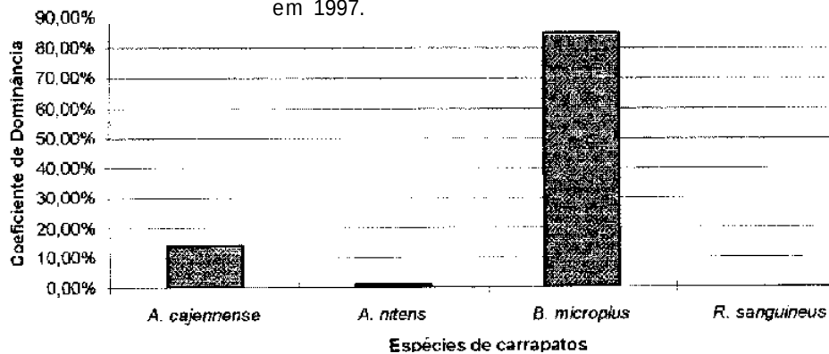
Gráfico 3: Coeficiente de Dominância entre espécies de carrapatos para Bos taurus examinados na Zona Fisiográfica de Resende, estado do Rio de Janeiro, em 1997.
