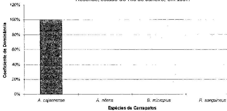
Gráfico 6: Coeficiente de Dominância entre espécies de carrapatos para Sus scrofa examinados na Zona Fisiográfica de Resende, estado do Rio de Janeiro, em 1997.
