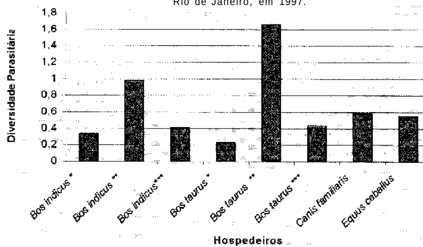
Gráfico 7: Diversidade Parasitária para quatro espécies de hospedeiros parasitados por mais de uma espécie de carrapato, na Zona Fisiográfica de Resende, estado do Rio de Janeiro, em 1997.
