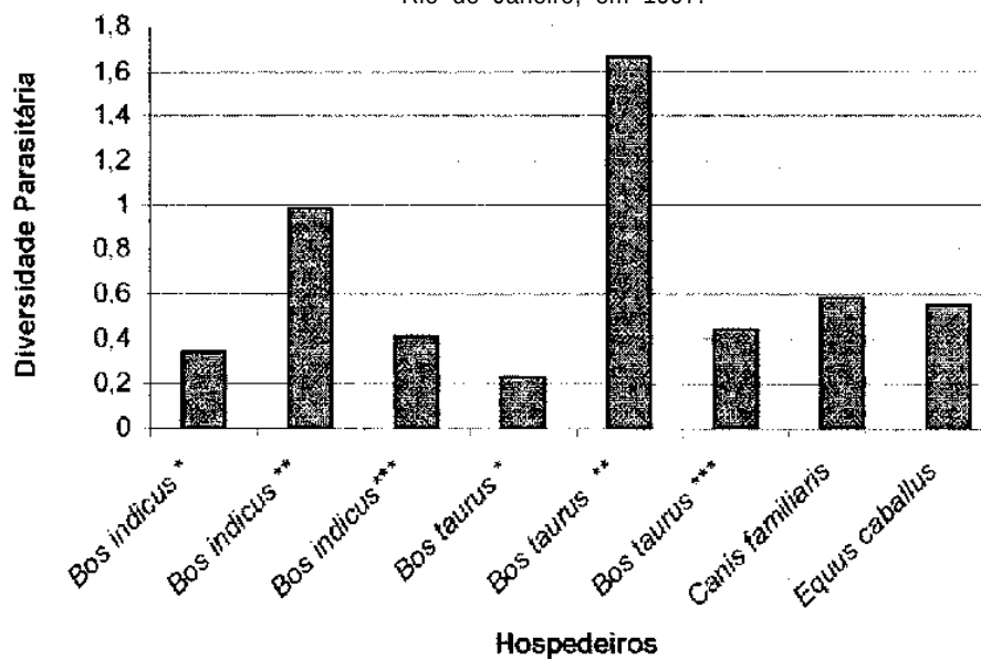
Gráfico 7: Diversidade Parasitária para quatro espécies de hospedeiros parasitados por mais de uma espécie de carrapato, na Zona Fisiográfica de Resende, estado do Rio de Janeiro, em 1997.
