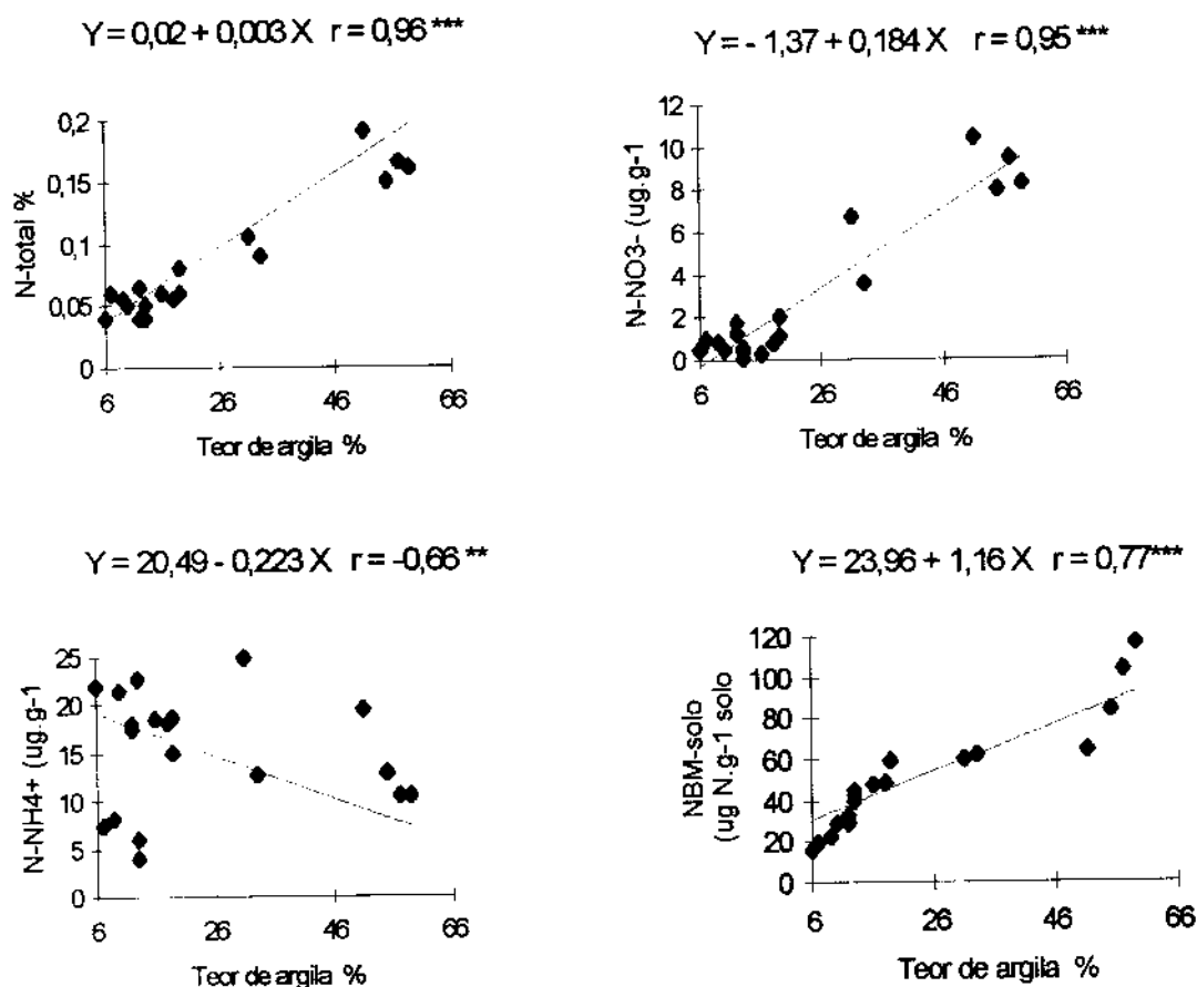
Figura 8. N-total, N-NO 3 - , N-NH 4 + e NBMS em função do teor de argila (média dos povoamentos nos Municípios).
