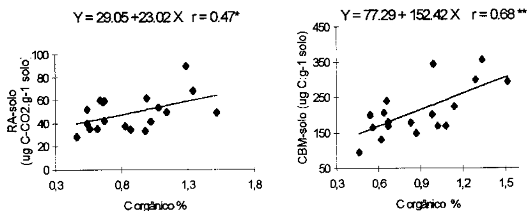
Figura 5. RA e CBM-solo em função do C orgânico do solo (média dos povoamentos nos Municípios).
