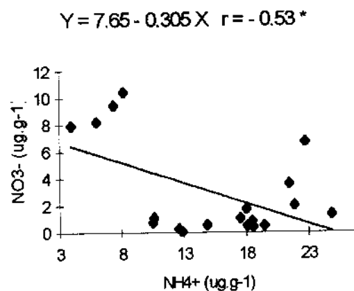
Figura 6. Teor de N-NO 3 - em função do teor de N-NH 4 + do solo (média dos povoamentos nos Municípios).
