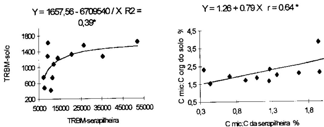
Figura 4. TRBM-solo em função da TRBM-serapilheira ( \mu\text{g C-CO}_2.\text{g}^{-1} \text{C microbiano.h}^{-1} ) e a relação C mic:C org do solo em função da relação C mic:C da serapilheira (média dos povoamentos nos Municípios).
