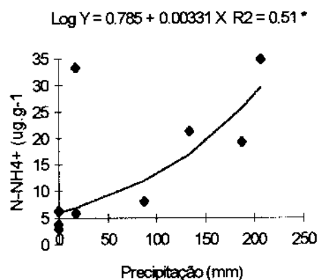
Figura 9. Teor de \text{N-NH}_4^+ no solo em função da precipitação mensal (média das épocas coletas por Município)
