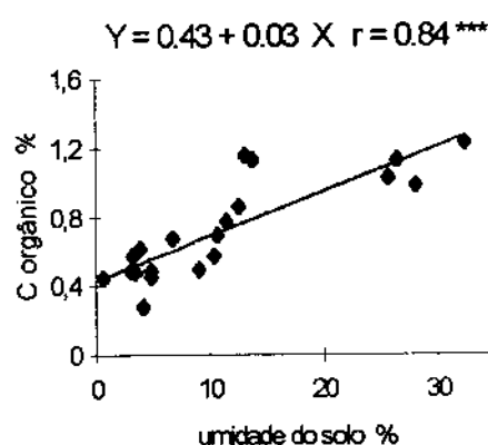
Figura 11. Carbono orgânico em função da umidade do solo (média dos povoamentos nos Municípios).
