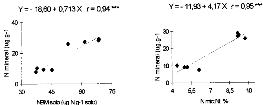
Figura 12. N mineral em função de NBM e Nmic:Nt do solo (média dos povoamentos por época de coleta)
