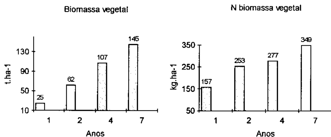
Figura 16. Produção e conteúdo de N da biomassa vegetal do eucalipto nas diferentes idades (média dos Municípios)
