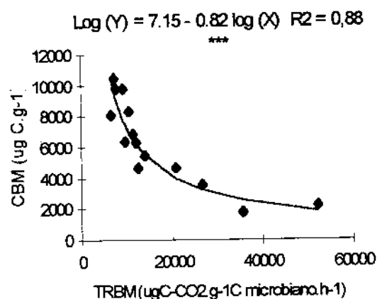
Figura 3. CBM-serapilheira em função da TRBM-serapilheira (média dos povoamentos nos Municípios).
