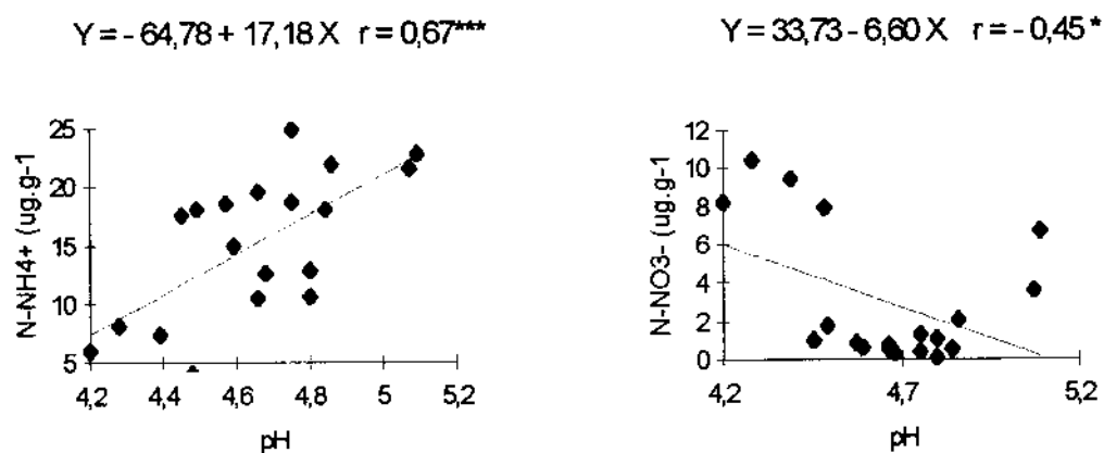
Figura 4. N-NH_4^+ , N-NO_3^- em função do pH do solo (média dos povoamentos nos Municípios).
