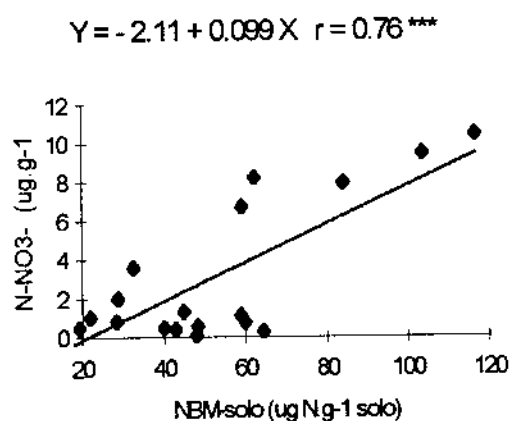
Figura 7. Teor de N-NH 4 + e N-NO 3 - em função do NBMS (média dos povoamentos nos Municípios).
