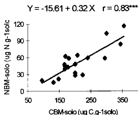
Figura 7. NBM-solo em função de CBM-solo (média dos povoamentos nos Municípios).
