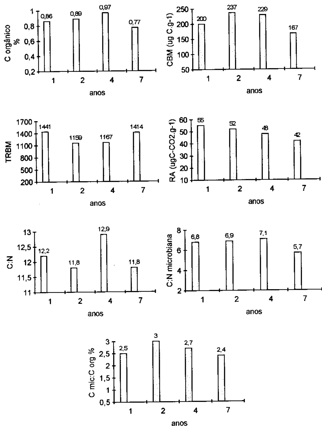
Figura 1. Carbono orgânico, C da biomassa microbiana, respiração acumulada, o índice TRBM ( \mu\text{g C-CO}_2 \cdot \text{g}^{-1} \text{C microbiano} \cdot \text{h}^{-1} ) e as relações C mic:C org, C:N microbiana e C:N dos solos sob eucalipto de diferentes idades (média dos povoamentos nos Municípios).
