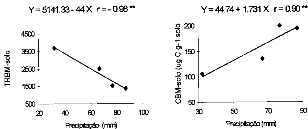
Figura 10. TRBM ( \mu\text{g C-CO}_2.\text{g}^{-1}\text{ C microbiano.h}^{-1} ) e CBM-solo de eucalipto de em função da precipitação mensal (média por época de coleta).
