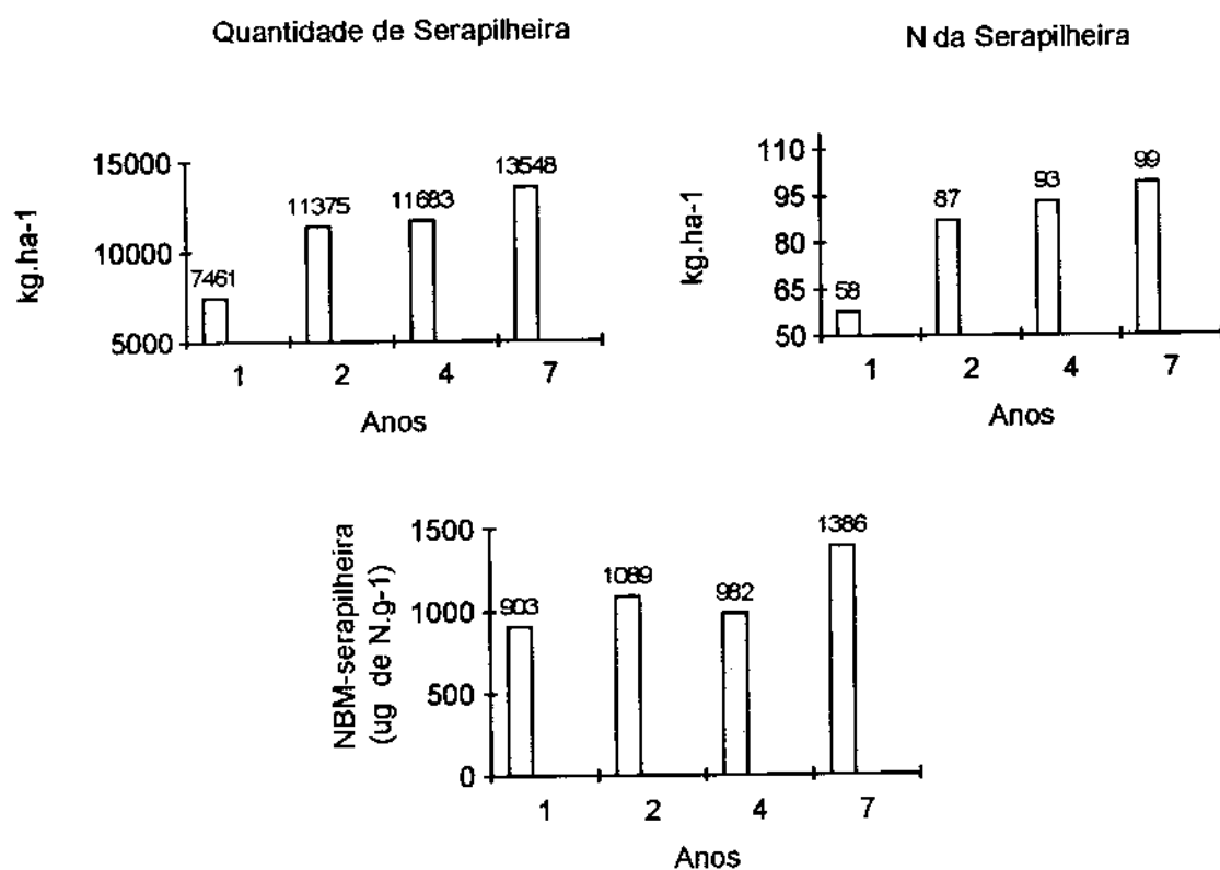
Figura 2. Quantidade de serapilheira e seu conteúdo de N e N da biomassa microbiana da serapilheira de eucalipto sob diferentes idades (média dos povoamentos nos Municípios).
