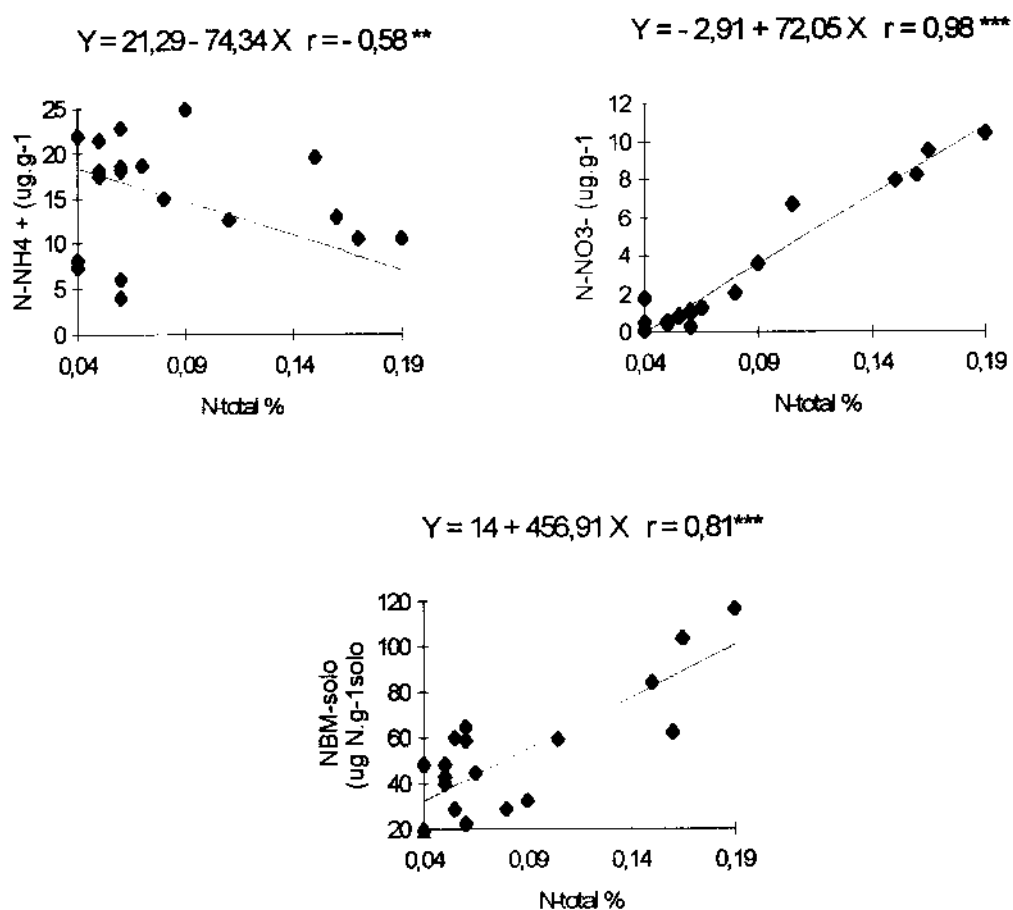
Figura 5. Valor de N-NH_4^+ , N-NO_3^- e NBMS em função do teor de N total do solo (média dos povoamentos nos Municípios).
