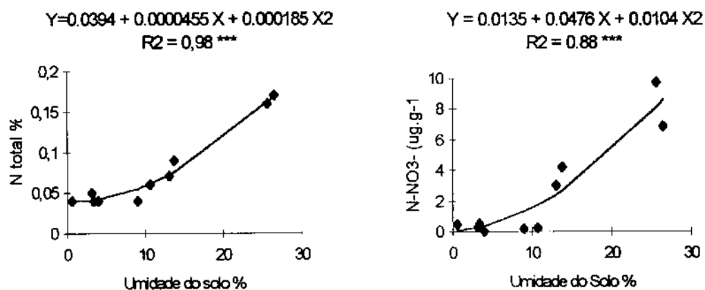
Figura 10. N-total e \text{N-NO}_3^- em função da umidade do solo (média das épocas coletas por Município)
