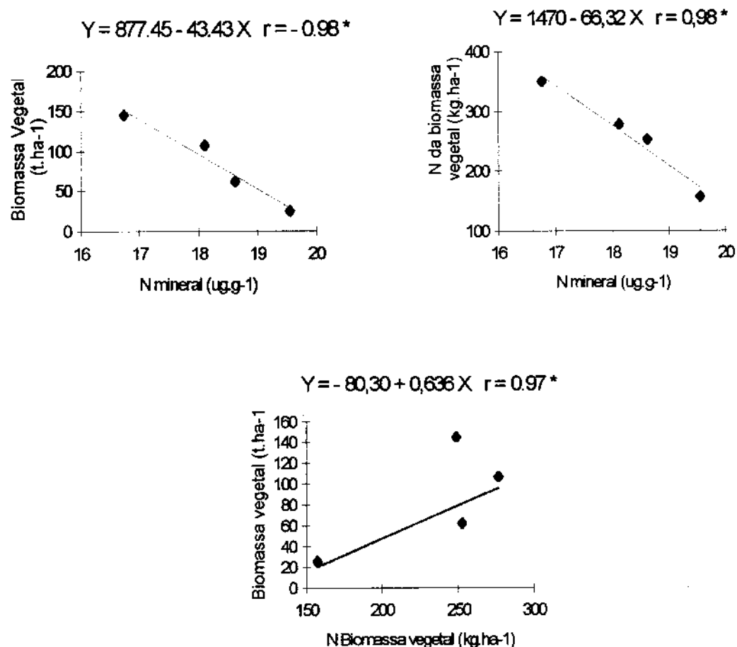
Figura 14. Biomassa Vegetal e N acumulado em função do N mineral, e produção de biomassa vegetal em função do N da biomassa Vegetal (média das idades)
