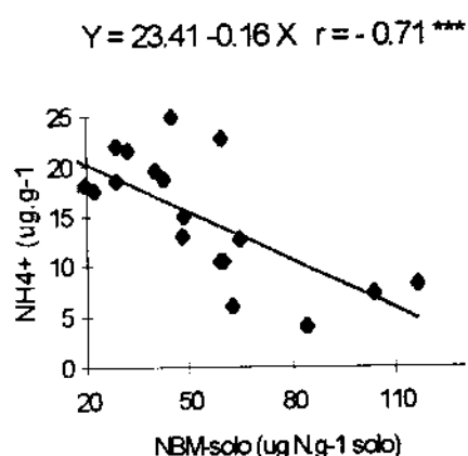
Figura 7. Teor de N-NH 4 + e N-NO 3 - em função do NBMS (média dos povoamentos nos Municípios).
