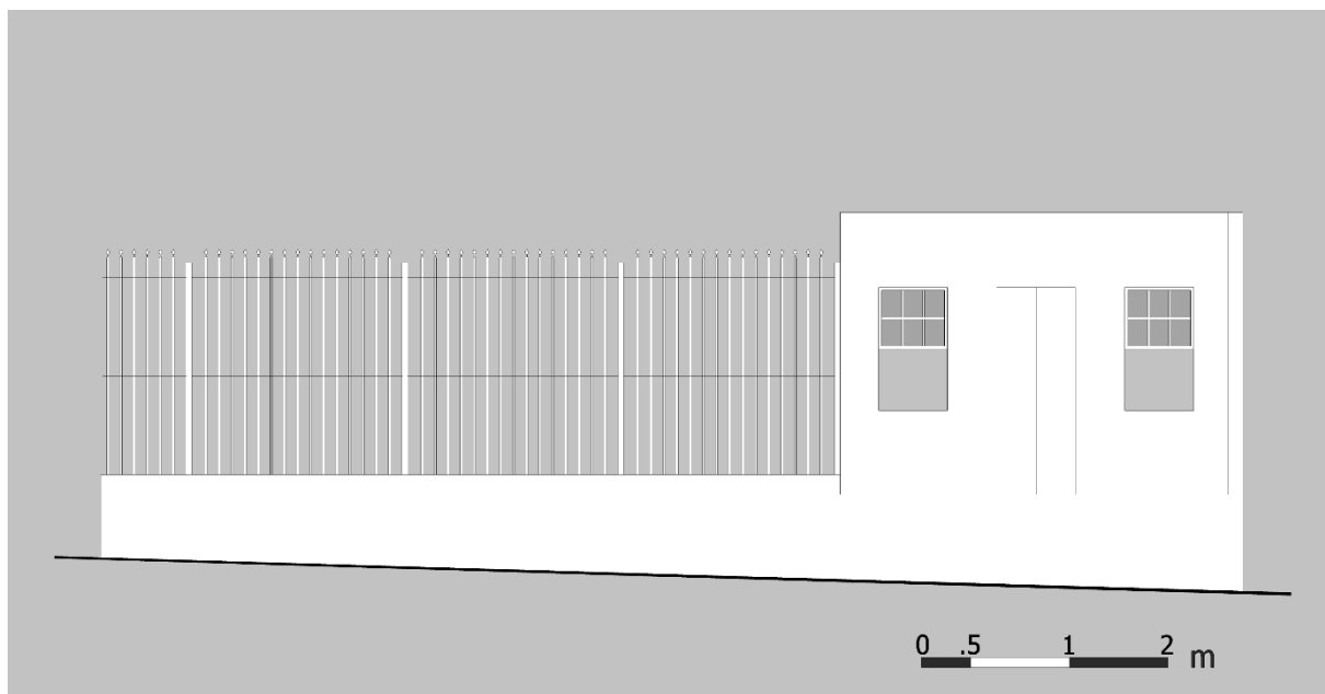
Fachada posterior
