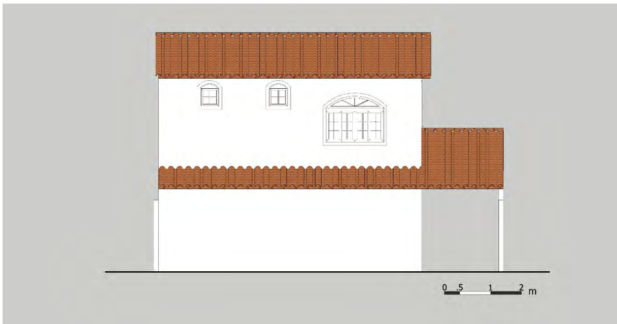
Fachada posterior
