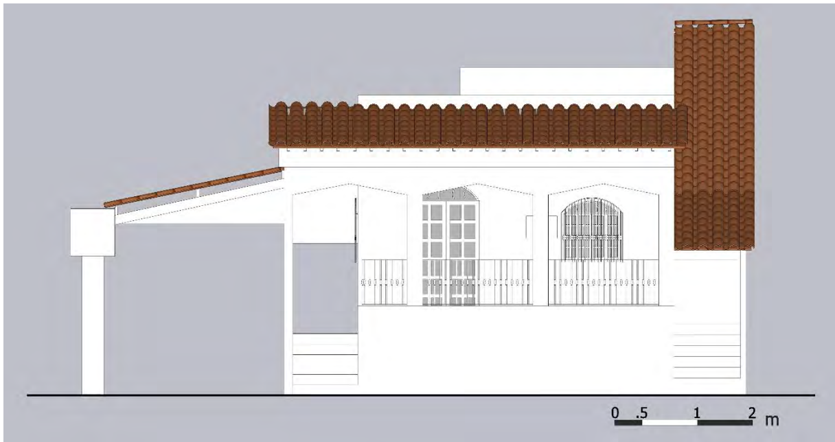
Fachada frontal
