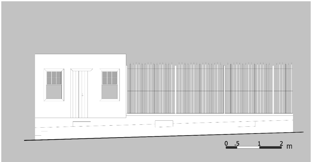
Fachada frontal
