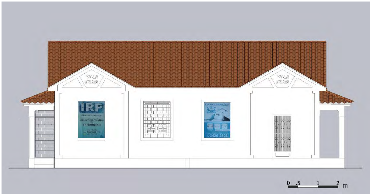
Fachada frontal
