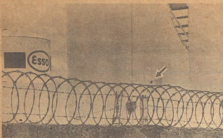
Corinto: Tanque de almacenamiento de químicos dañado por el charnel de una bomba.
